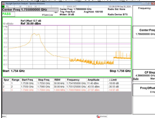
Band Edge_Band4_10MHz_PUSCH_1750MHz_Chain0
