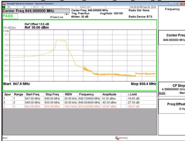
Band5_3MHz_Chain0_847.5MHz_NBI_1_QPSK_6_0
