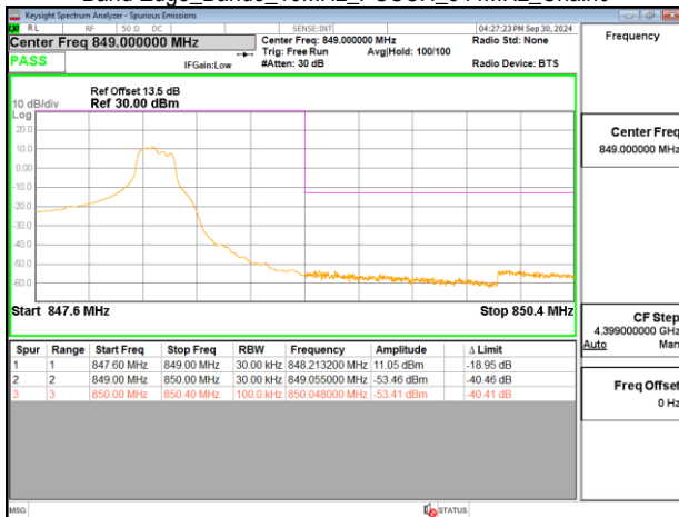
Band Edge_Band5_10MHz_PUSCH_844MHz_Chain0
