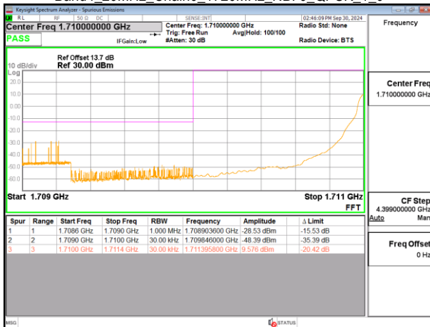
Band4_20MHz_Chain0_1720MHz_NBI 0_QPSK 1 0
