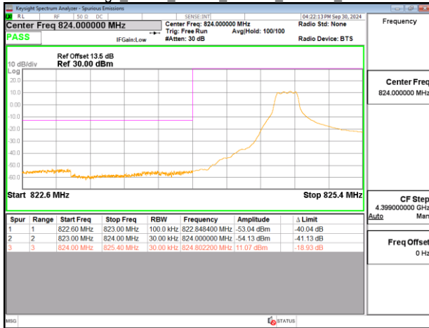
Band Edge_Band5_10MHz_PUSCH_829MHz_Chain0
