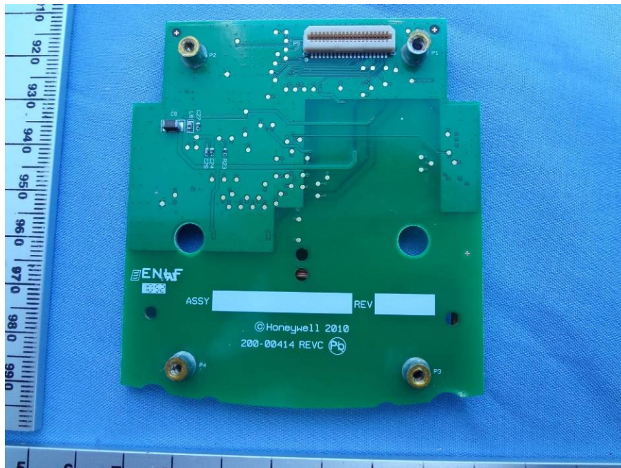
125 KHz HID eProx MCM 4025A RF Module Front Side
