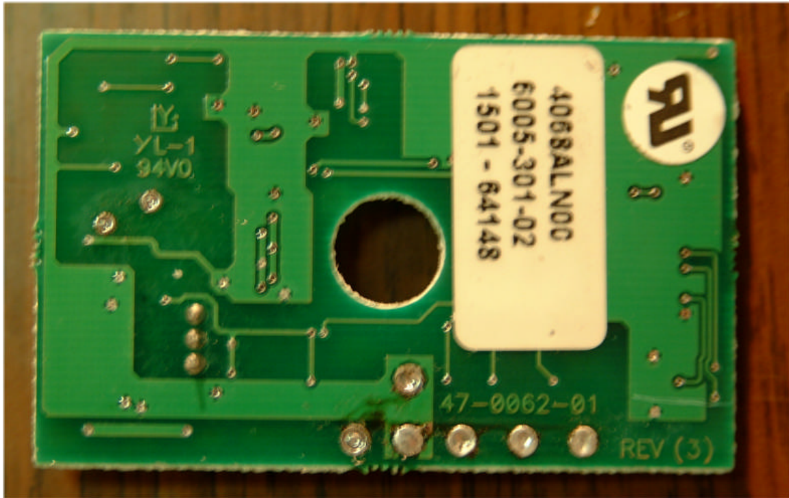
FIG8-8 4068 module side 1
