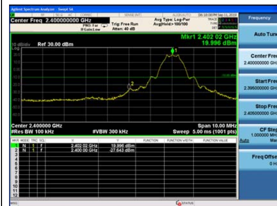
BLE V5.0-2M, Channel No.: 0
