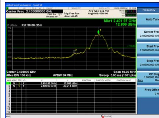
BLE V5.0-125K, Channel No.: 0
