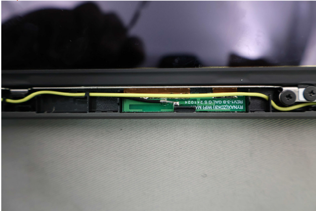
BT&amp;WIFI_Antenna(1)
