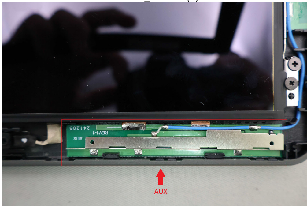
WWAN_Antenna(1)
