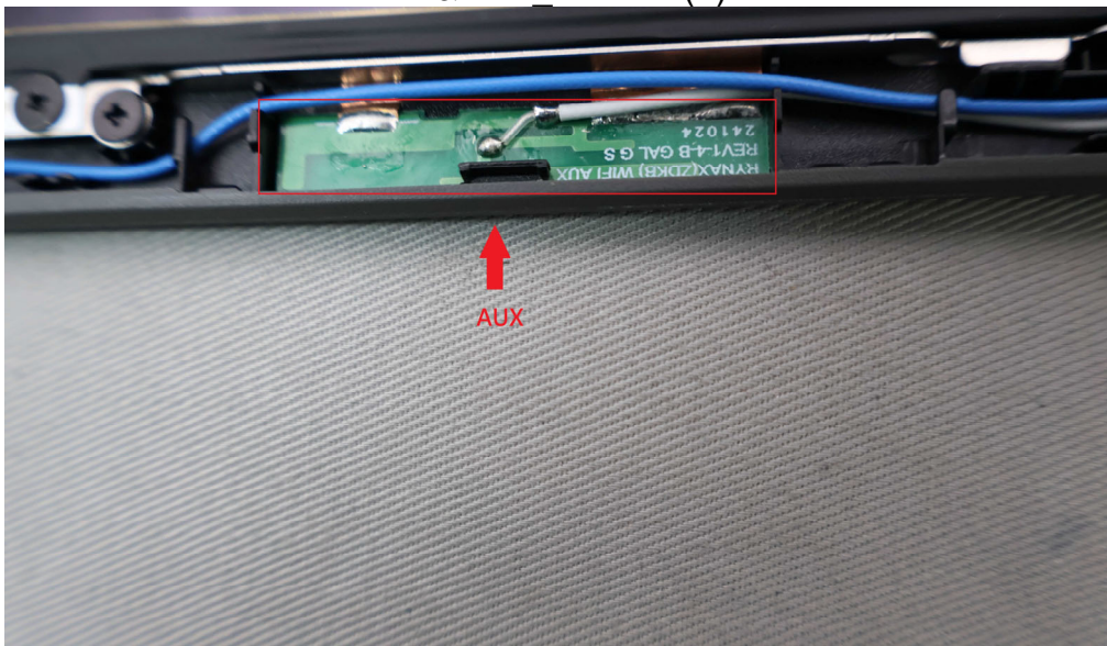
BT&amp;WIFI_Antenna(1)
