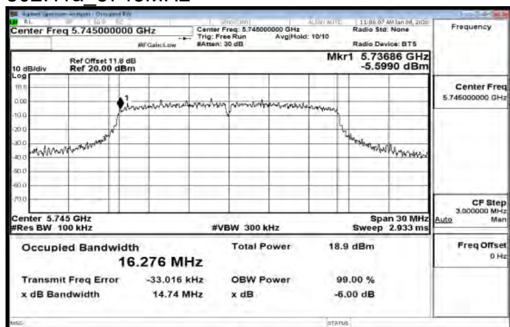
802.11a 5745MHz
