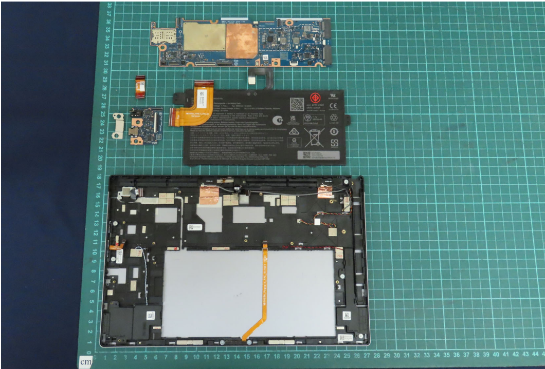
(24) EUT Photo
