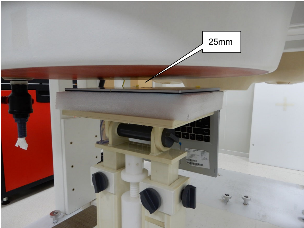
EUT Back(NB)
