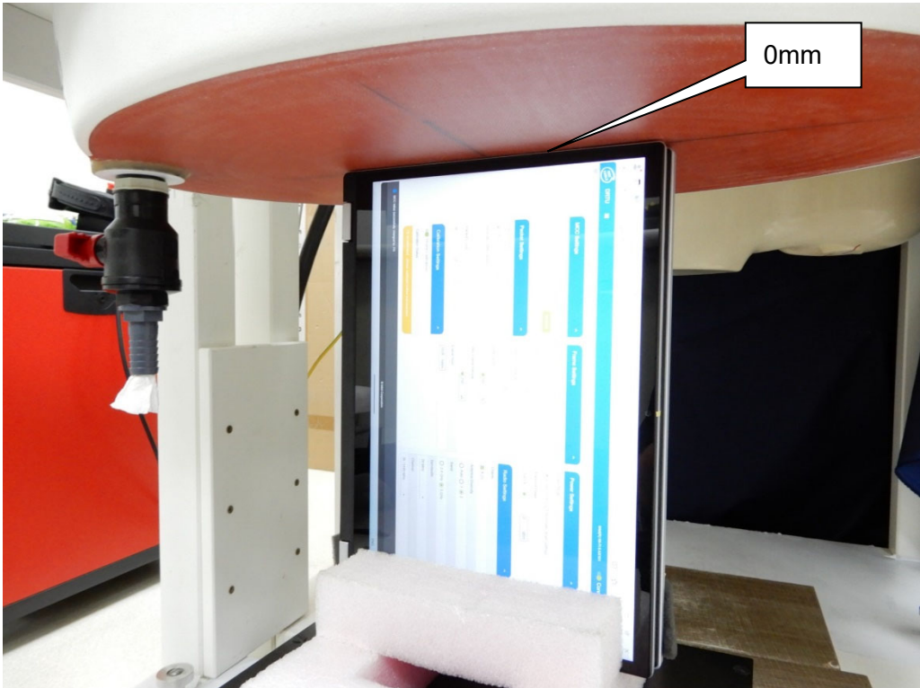
EUT Left-side(PAD)
