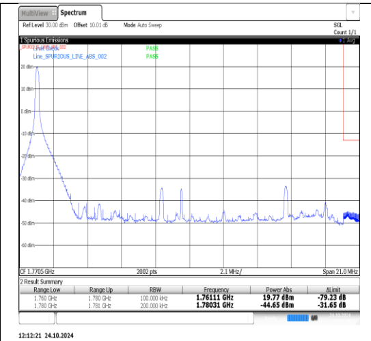
Band66-20MHz-QPSK-132572-1RB#99-PASS
