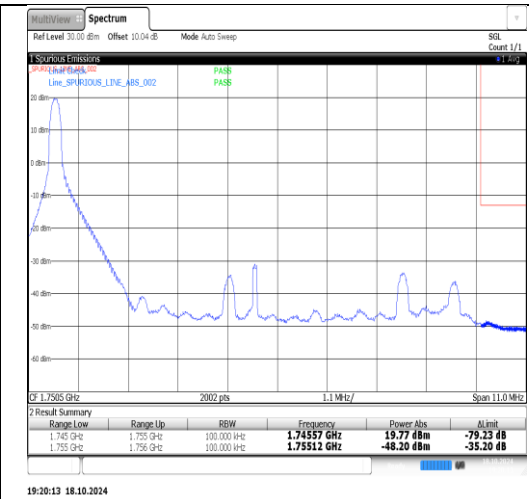
Band4-10MHz-QPSK-20350-1RB#49-PASS
