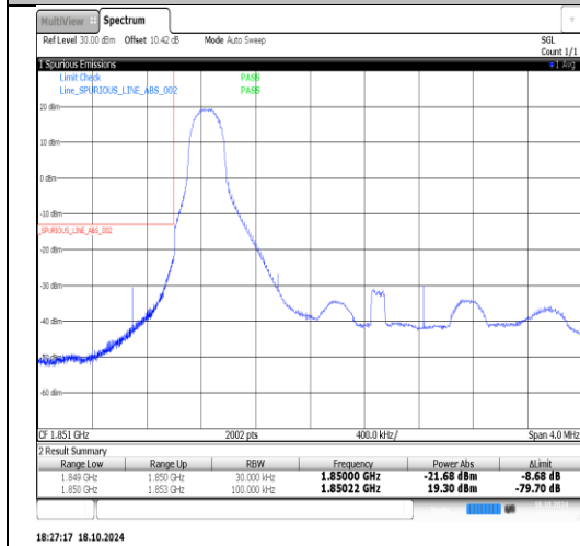
Band2-3MHz-16QAM-18615-1RB#14-PASS
