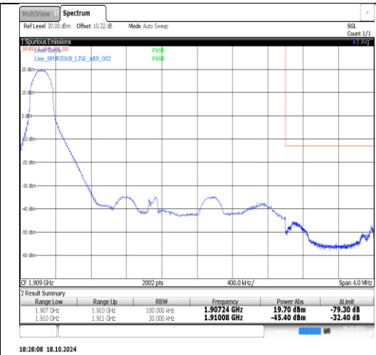
Band2-3MHz-QPSK-19185-1RB#14-PASS
