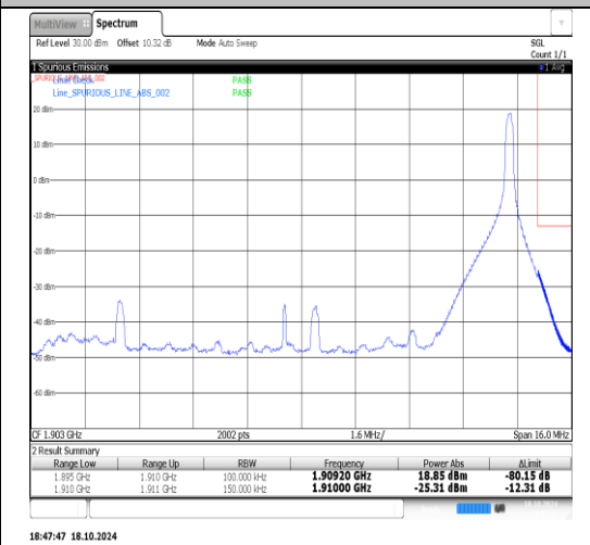
Band2-20MHz-QPSK-18700-100RB#0-PASS
