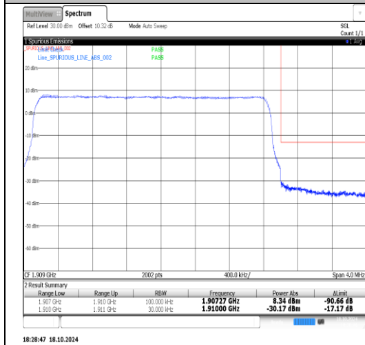
Band2-3MHz-QPSK-19185-1RB#14-PASS
