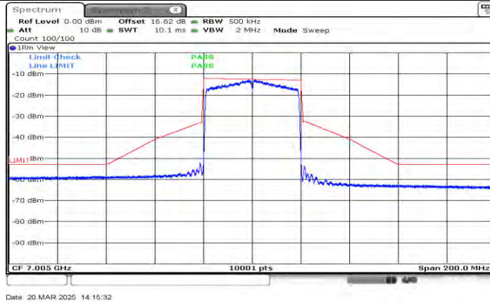
11AX40MIMO_Ant1_7005
