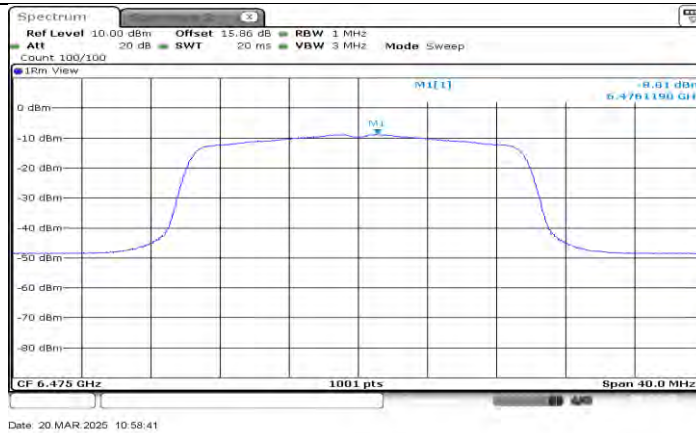
11AX20MIMO_Ant2_6475
