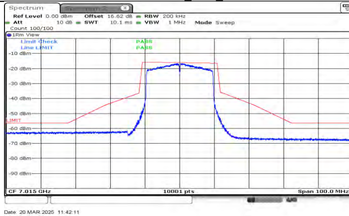
11AX20MIMO_Ant1_7015
