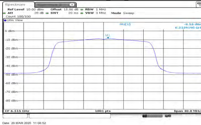
11AX20MIMO_Ant2_6515
