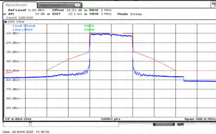
11AX80MIMO_Ant1_6865
