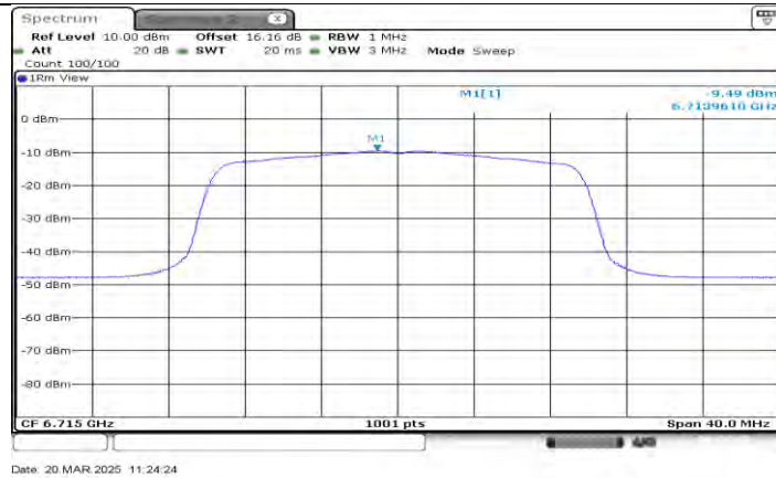
11AX20MIMO_Ant2_6715
