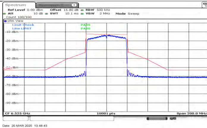
11AX40MIMO_Ant1_6525
