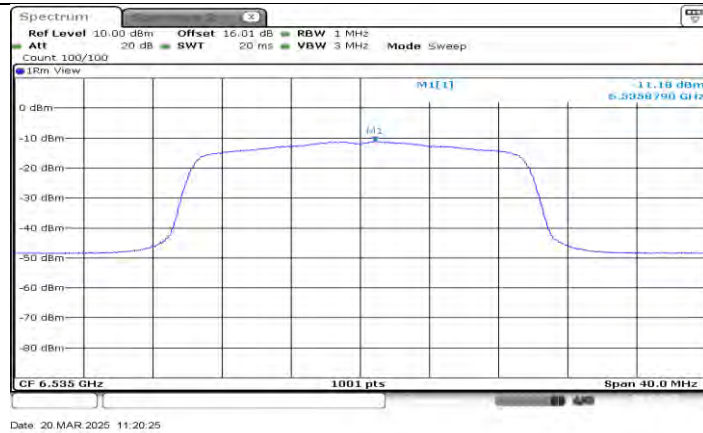
11AX20MIMO_Ant1_6535
