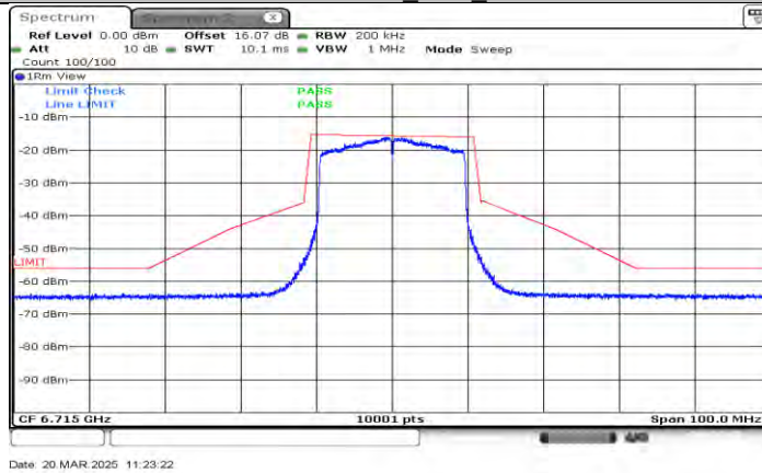
11AX20MIMO_Ant1_6715
