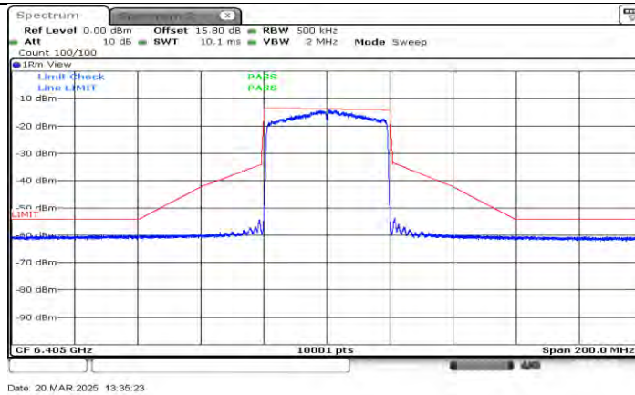
11AX40MIMO_Ant1_6405
