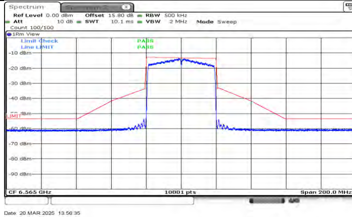
11AX40MIMO_Ant1_6565
