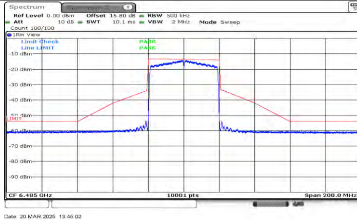
11AX40MIMO_Ant1_6485
