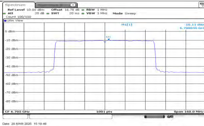
11AX80MIMO_Ant1_6705
