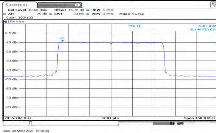
11AX80MIMO_Ant1_6785
