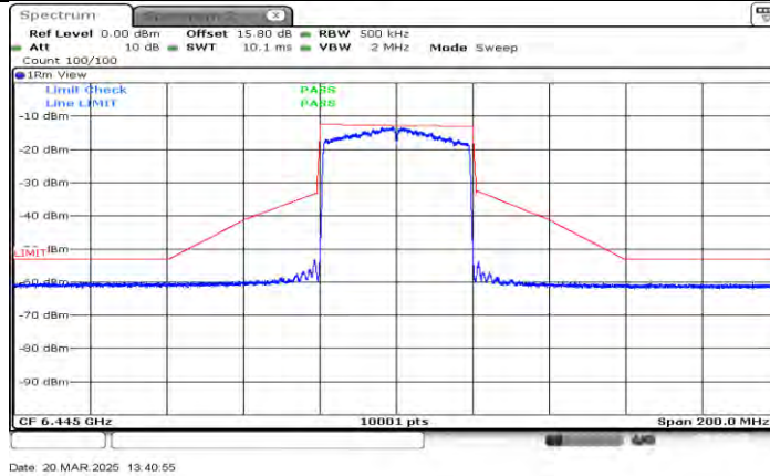
11AX40MIMO_Ant1_6445
