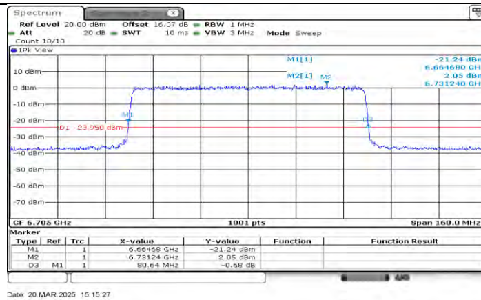
11AX80MIMO_Ant1_6705
