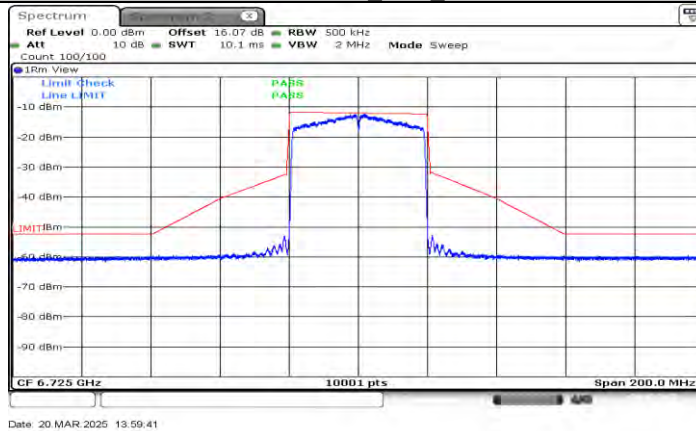
11AX40MIMO_Ant1_6725
