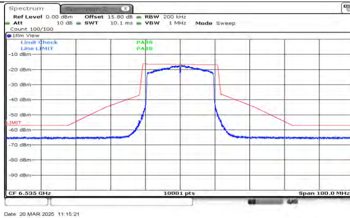
11AX20MIMO_Ant1_6535
