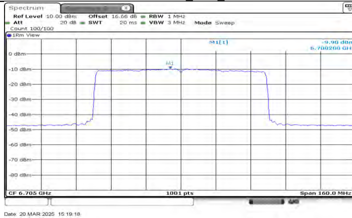
11AX80MIMO_Ant2_6705
