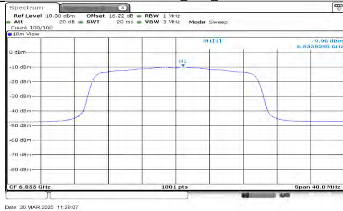
11AX20MIMO_Ant1_6855
