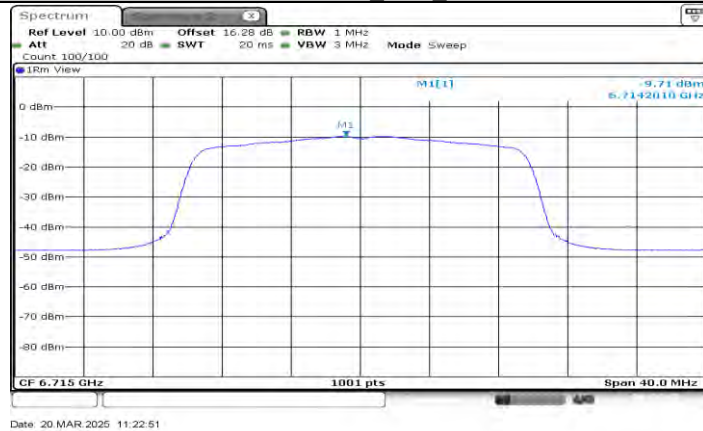
11AX20MIMO_Ant1_6715
