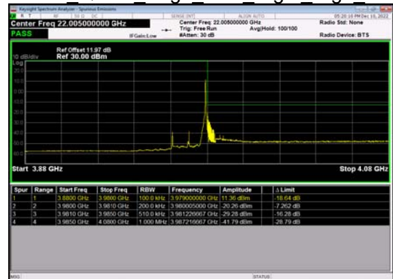
N77(20M)_DFT-s- OFDM QPSK Edge 1RB Right High CH
