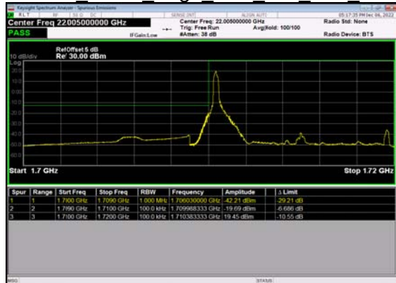
N66(10M)_DFT-s- OFDM BPSK Edge 1RB Left Low CH
