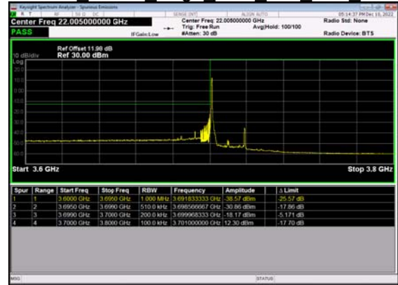
N77(20M)_DFT-s- OFDM QPSK Edge 1RB Left Low CH
