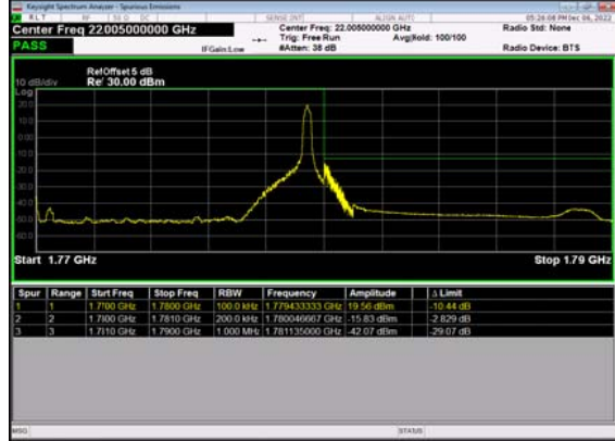
N66(20M)_DFT-s- OFDM BPSK Edge 1RB Right High CH
