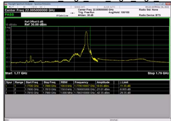
N66(15M)_DFT-s- OFDM QPSK Edge 1RB Right High CH
