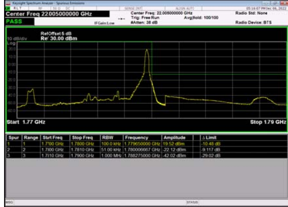
N66(5M)_DFT-s- OFDM BPSK Edge 1RB Right High CH
