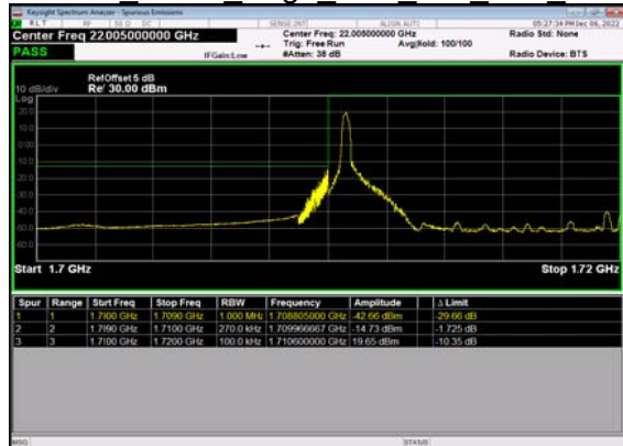
N66(25M)_DFT-s- OFDM BPSK Edge 1RB Left Low CH
