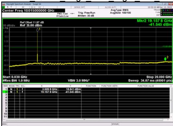
N77(20M)_DFT-s- OFDM QPSK Edge 1RB Right Mid CH
