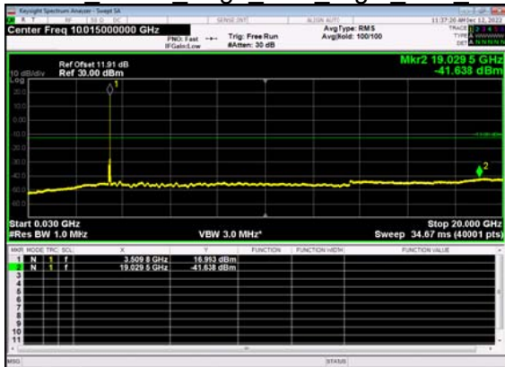
N77(60M)_DFT-s- OFDM QPSK Edge 1RB Right Low CH
