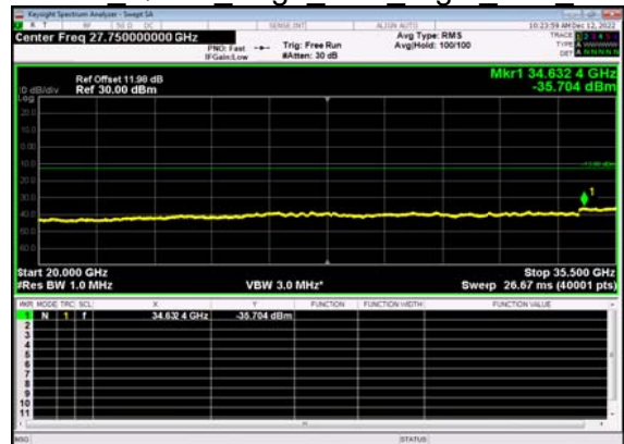
N77(20M)_DFT-s- OFDM QPSK Edge 1RB Right Low CH
