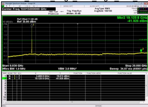
N77(20M)_DFT-s- OFDM QPSK Edge 1RB Right Low CH
