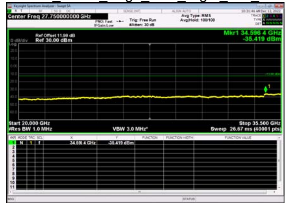
N77(20M)_DFT-s- OFDM BPSK Edge 1RB Right Mid CH
