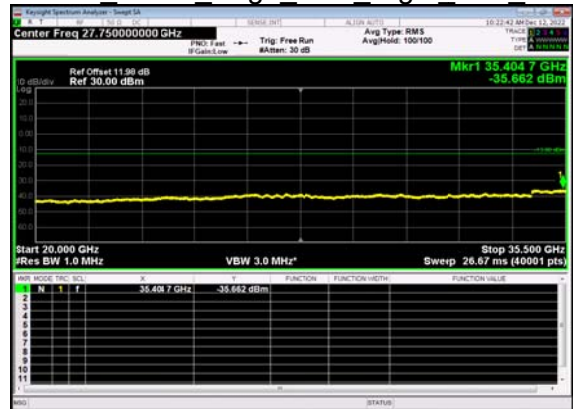
N77(20M)_DFT-s- OFDM BPSK Edge 1RB Right Low CH
