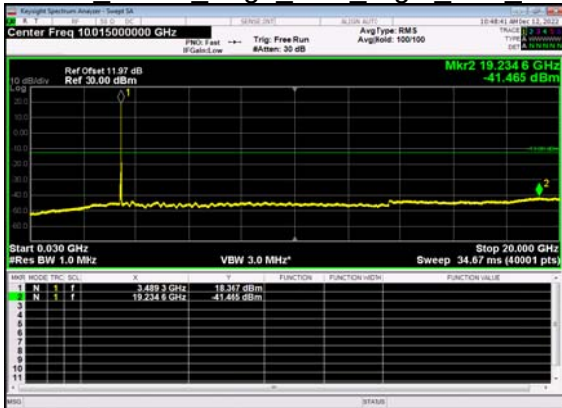
N77(40M)_DFT-s- OFDM QPSK Edge 1RB Right Low CH
