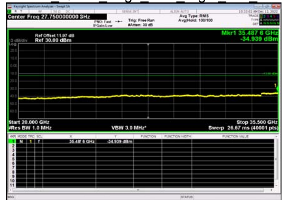
N77(20M)_DFT-s- OFDM QPSK Edge 1RB Right Mid CH
