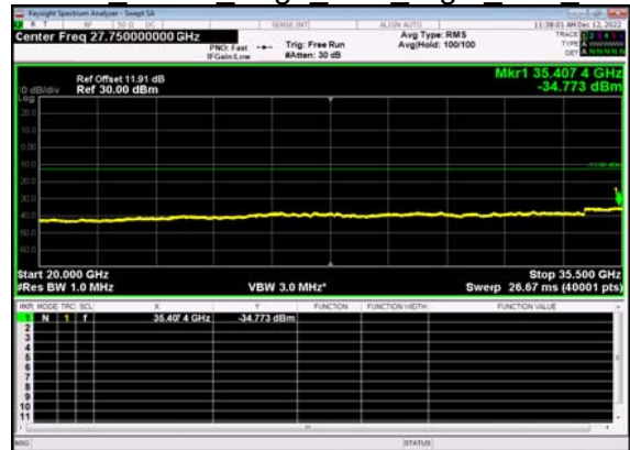
N77(60M)_DFT-s- OFDM QPSK Edge 1RB Right Low CH
