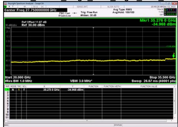
N77(40M)_DFT-s- OFDM QPSK Edge 1RB Right Low CH
