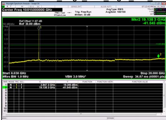
N77(15M)_DFT-s- OFDM BPSK Edge 1RB Right Mid CH
