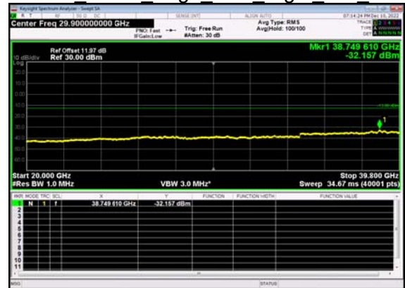
N77(15M)_DFT-s- OFDM BPSK Edge 1RB Right Mid CH
