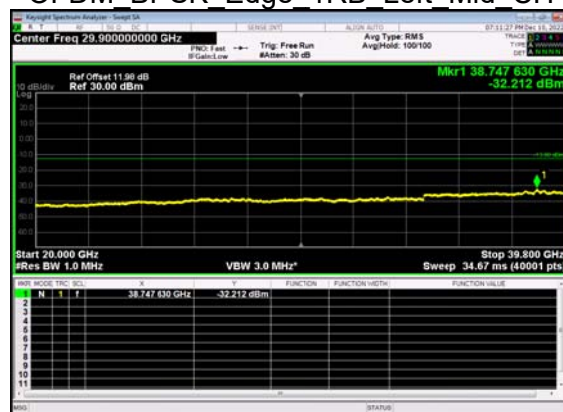
N77(15M)_DFT-s- OFDM BPSK Edge 1RB Left Mid CH
