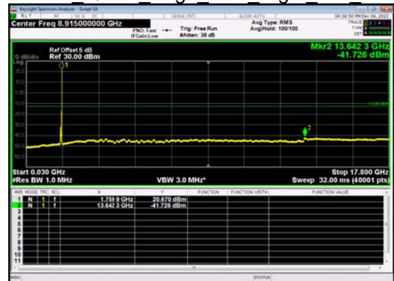
N66(30M)_DFT-s- OFDM QPSK Edge 1RB Right Mid CH
