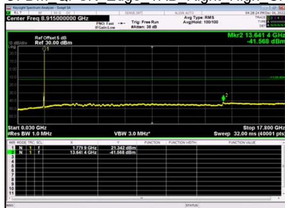
N66(25M)_DFT-s- OFDM QPSK Edge 1RB Right High CH
