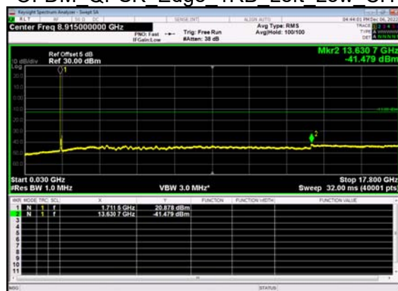
N66(40M)_DFT-s- OFDM QPSK Edge 1RB Left Low CH
