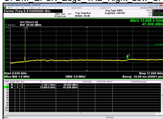
N66(40M)_DFT-s- OFDM QPSK Edge 1RB Right Low CH
