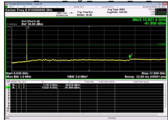
N66(10M)_DFT-s- OFDM QPSK Edge 1RB Left Mid CH
