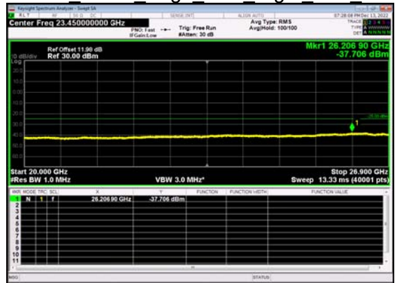
N41(100M)_DFT-s-OFDM BPSK Edge 1RB Right Low CH
