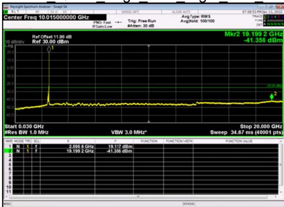
N41(100M)_DFT-s-OFDM QPSK Edge 1RB Right Low CH
