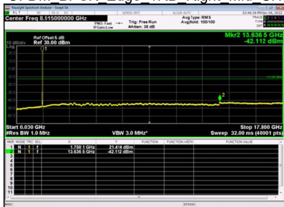
N66(10M)_DFT-s- OFDM BPSK Edge 1RB Right Mid CH
