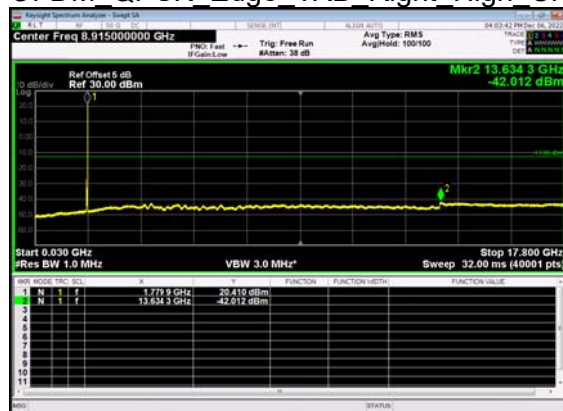
N66(15M)_DFT-s- OFDM QPSK Edge 1RB Right High CH
