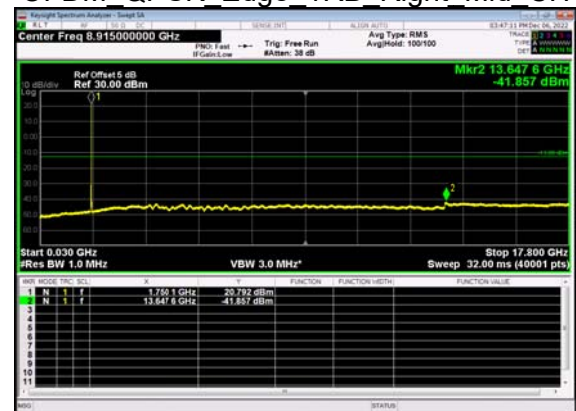
N66(10M)_DFT-s- OFDM QPSK Edge 1RB Right Mid CH
