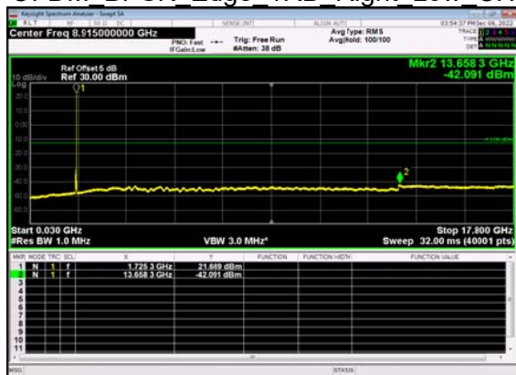
N66(15M)_DFT-s- OFDM BPSK Edge 1RB Right Low CH
