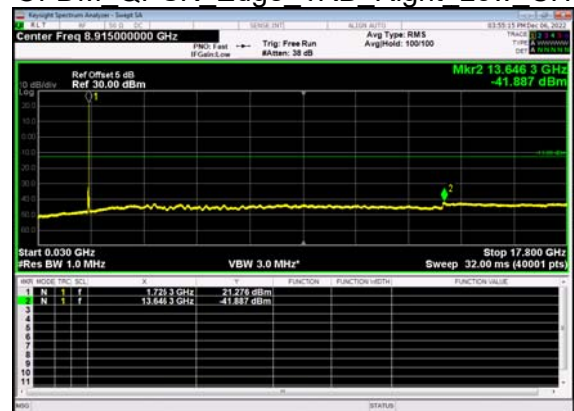
N66(15M)_DFT-s- OFDM QPSK Edge 1RB Right Low CH
