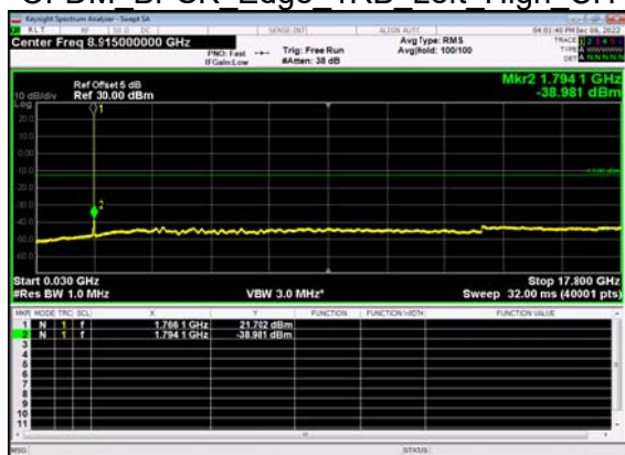
N66(15M)_DFT-s- OFDM BPSK Edge 1RB Left High CH
