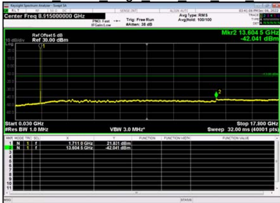
N66(10M)_DFT-s- OFDM BPSK Edge 1RB Left Low CH
