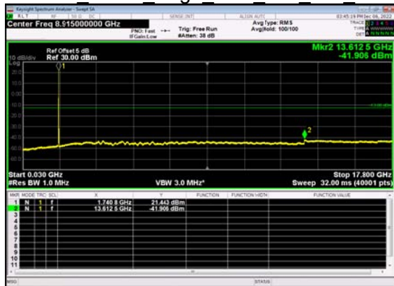
N66(10M)_DFT-s- OFDM BPSK Edge 1RB Left Mid CH
