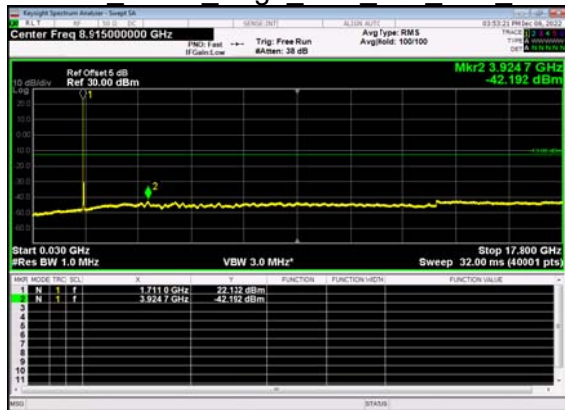
N66(15M)_DFT-s- OFDM BPSK Edge 1RB Left Low CH
