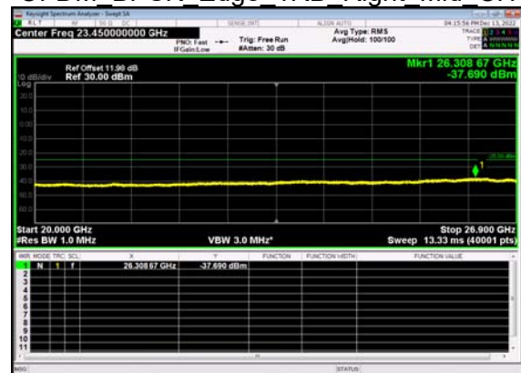
N41(15M)_DFT-s- OFDM BPSK Edge 1RB Right Mid CH
