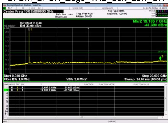
N41(15M)_DFT-s- OFDM BPSK Edge 1RB Left Low CH
