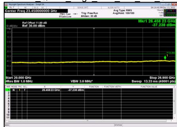
N41(15M)_DFT-s- OFDM QPSK Edge 1RB Left Mid CH
