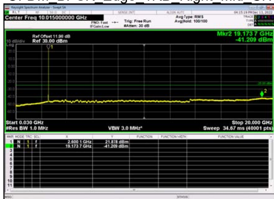
N41(15M)_DFT-s- OFDM BPSK Edge 1RB Right Mid CH
