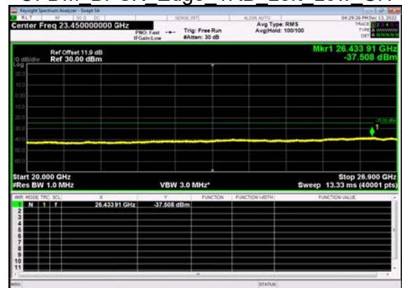
N41(20M)_DFT-s- OFDM BPSK Edge 1RB Left Low CH
