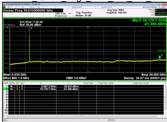
N41(15M)_DFT-s- OFDM QPSK Edge 1RB Left Mid CH
