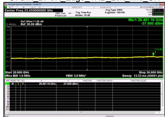
N41(15M)_DFT-s- OFDM BPSK Edge 1RB Left Mid CH
