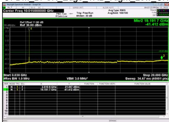
N41(15M)_DFT-s- OFDM BPSK Edge 1RB Right Low CH
