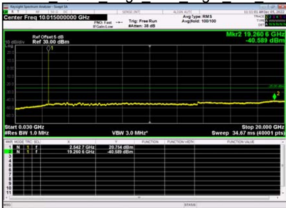
N7(15M)_DFT-s- OFDM QPSK Edge 1RB Right Mid CH
