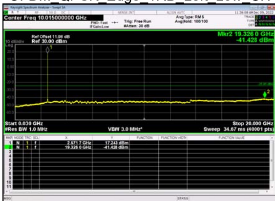
N38(15M)_DFT-s-OFDM QPSK Edge 1RB Left Low CH
