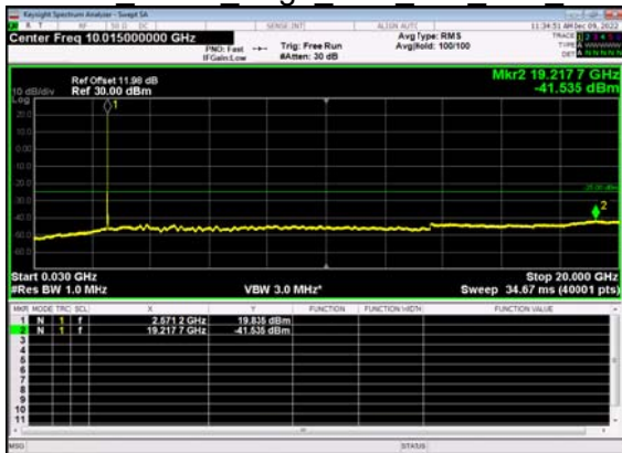
N38(15M)_DFT-s-OFDM BPSK Edge 1RB Left Low CH
