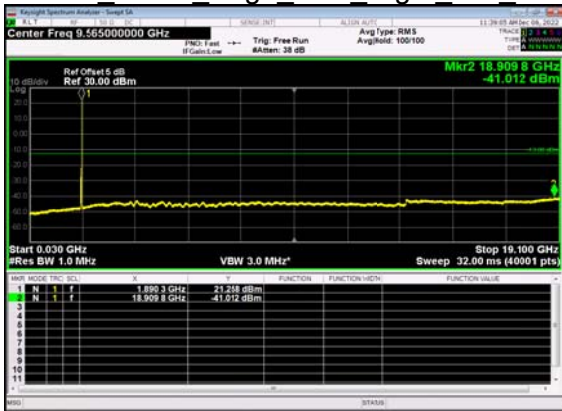
N2(20M)_DFT-s- OFDM BPSK Edge 1RB Right Mid CH
