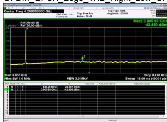
N5(20M)_DFT-s- OFDM QPSK Edge 1RB Right Low CH
