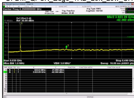
N5(20M)_DFT-s- OFDM QPSK Edge 1RB Left Low CH
