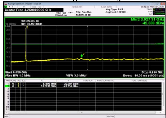
N5(15M)_DFT-s- OFDM QPSK Edge 1RB Right Low CH
