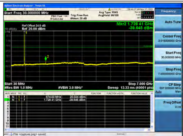
Band71 / 15MHz / Mid CH / 64QAM
