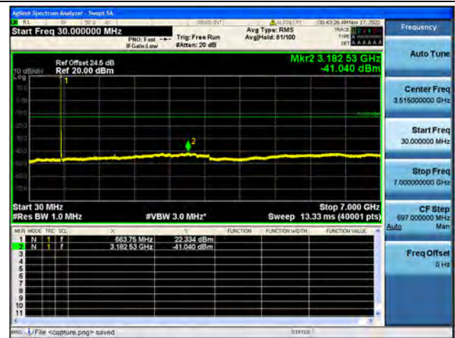
Band71 / 10MHz / Low CH / QPSK
