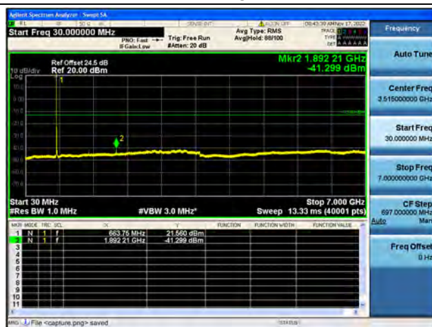
Band71 / 10MHz / Low CH / 16QAM
