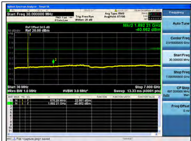
Band71 / 10MHz / Mid CH / QPSK
