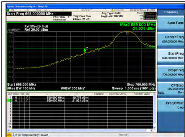
Band12 / 10MHz / Low CH / QPSK / 1 RB
