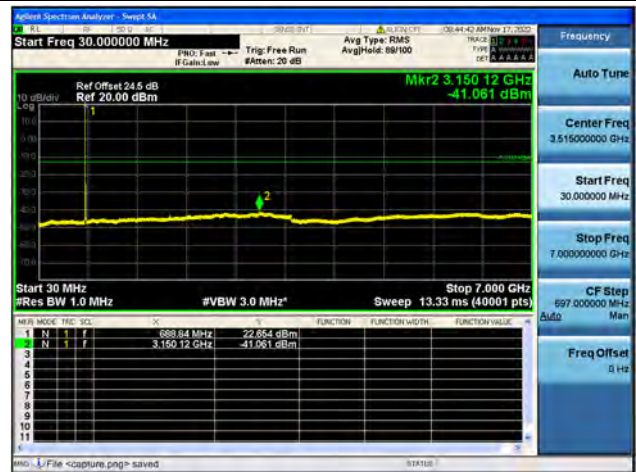
Band71 / 10MHz / High CH / QPSK
