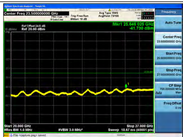
Band41-20G-27G / 5MHz / Low CH / 64QAM
