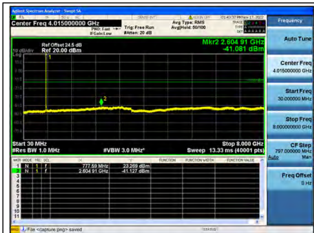
Band13 / 5MHz / Low CH / QPSK
