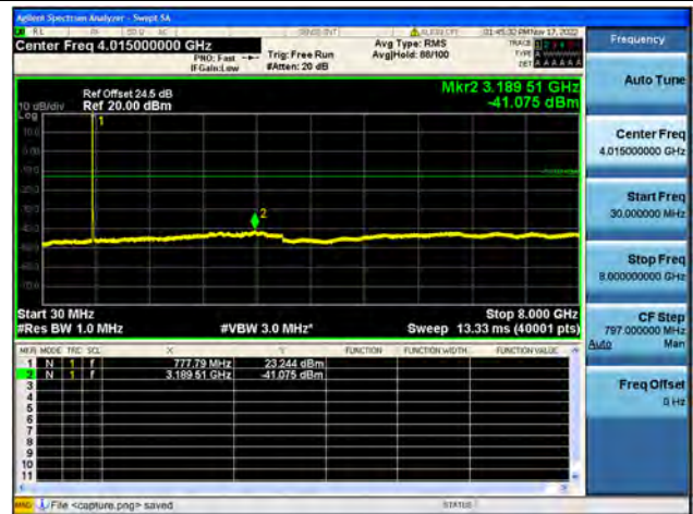
Band13 / 10MHz / Low CH / QPSK
