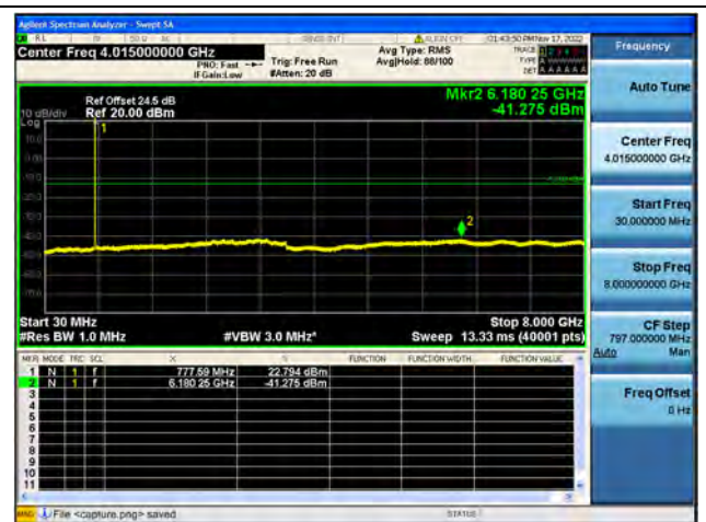
Band13 / 5MHz / Low CH / 16QAM
