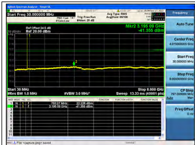
Band12 / 10MHz / Mid CH / QPSK
