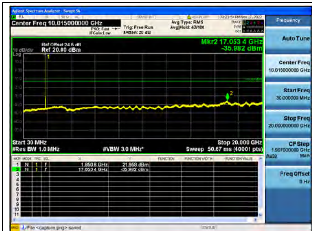
Band25 / 15MHz / Low CH / QPSK
