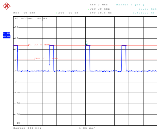
835MHz - GSM
