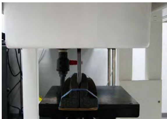
Fig.5 EUT Left Edge to flat phantom
