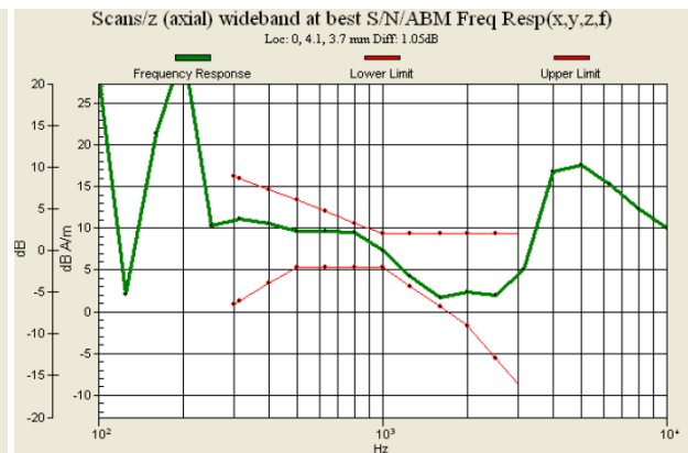
Fig. 9.2 GSM850 Ch189
