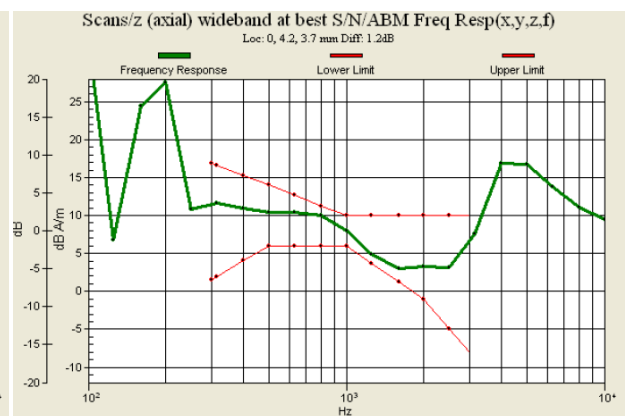
Fig. 9.6 GSM1900 Ch810
