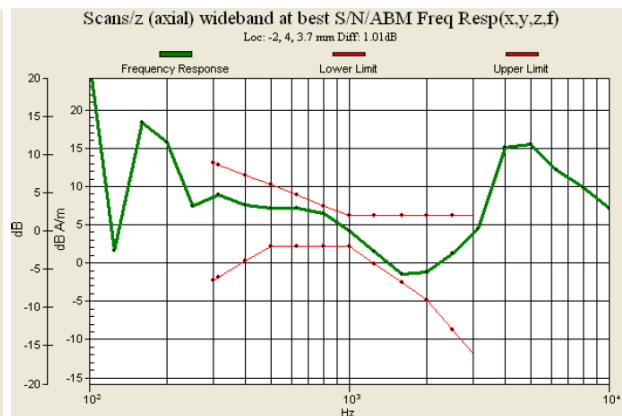
Fig. 9.2 WCDMA Band V Ch4182
