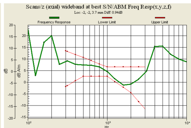
Fig. 9.4 WCDMA Band II Ch9262
