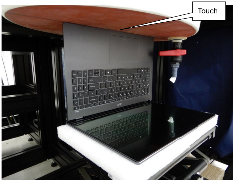
EUT Edge(Front)
