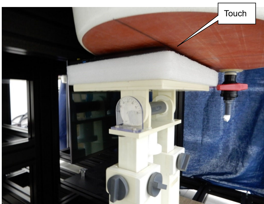
EUT Bottom
