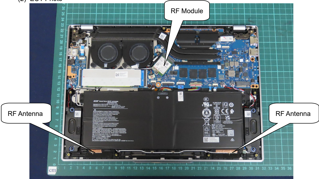
(2) EUT Photo
