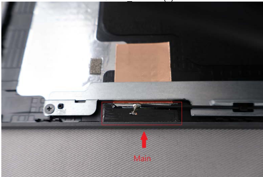
BT&WIFI Antenna(2)
