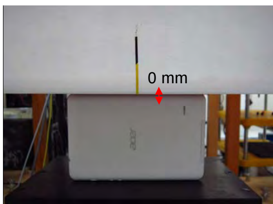
Fig.5 EUT Edge 3 to flat phantom
