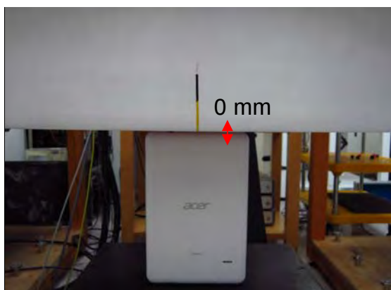
Fig.4 EUT Edge 1 to flat phantom
