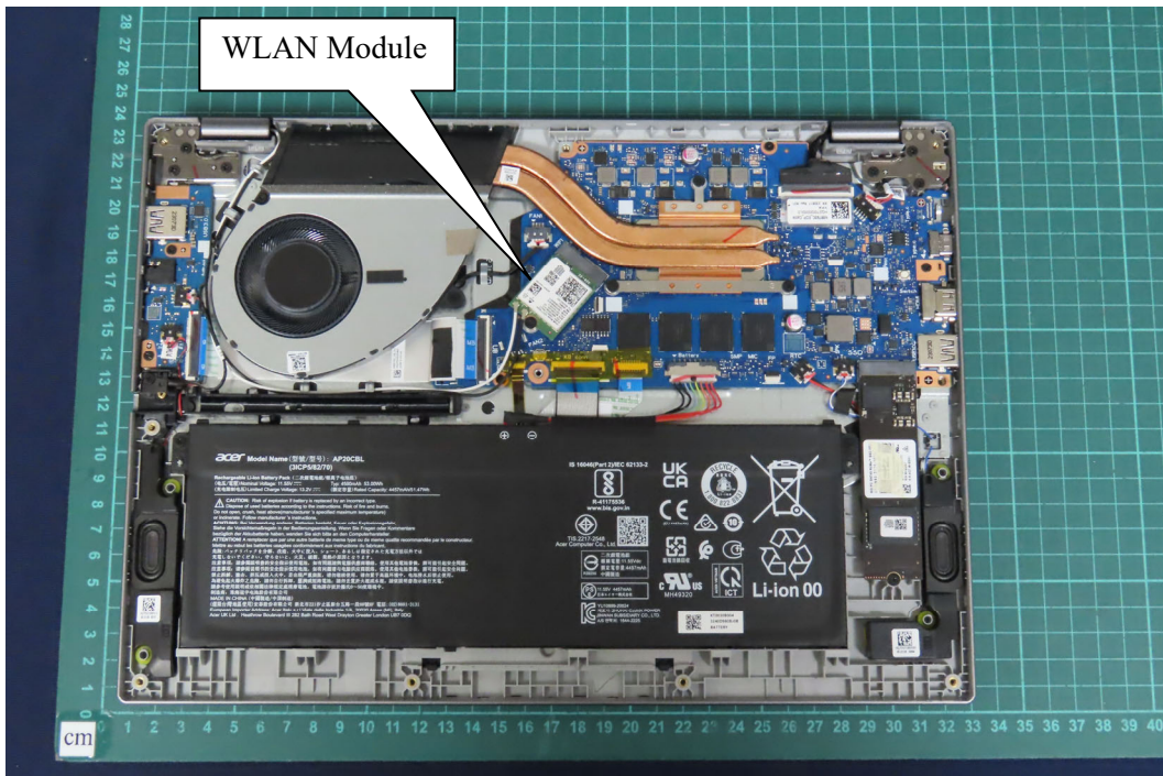
(4) EUT Photo
