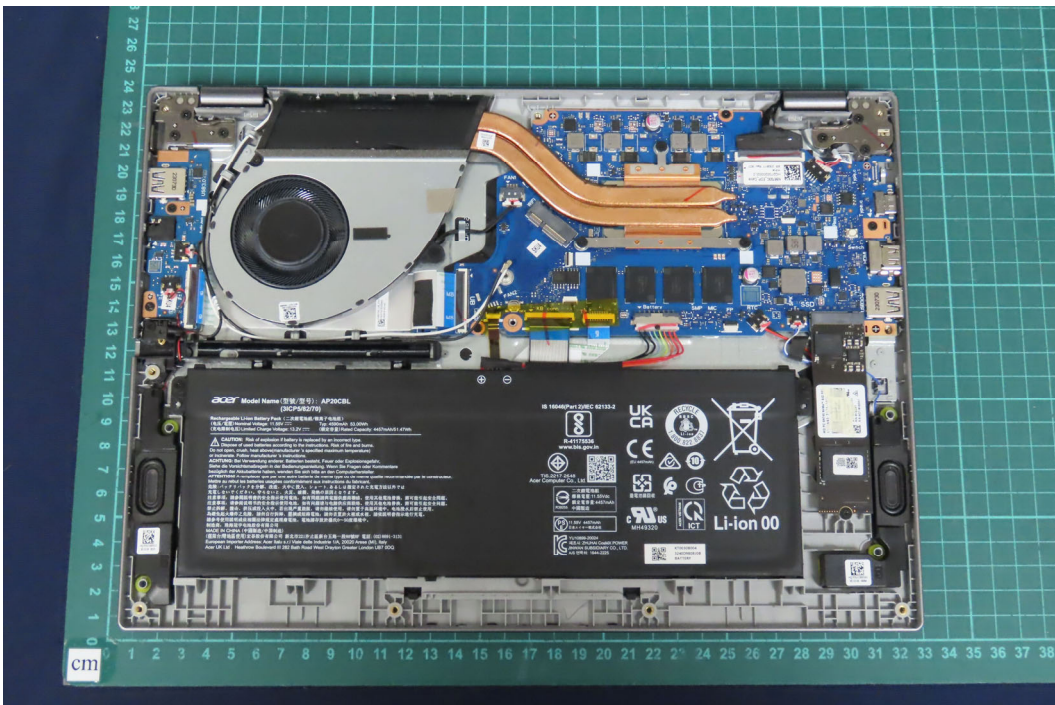
(8) EUT Photo
