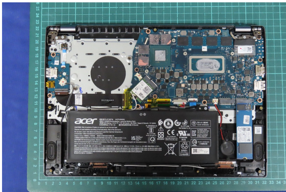
(12) EUT Photo
