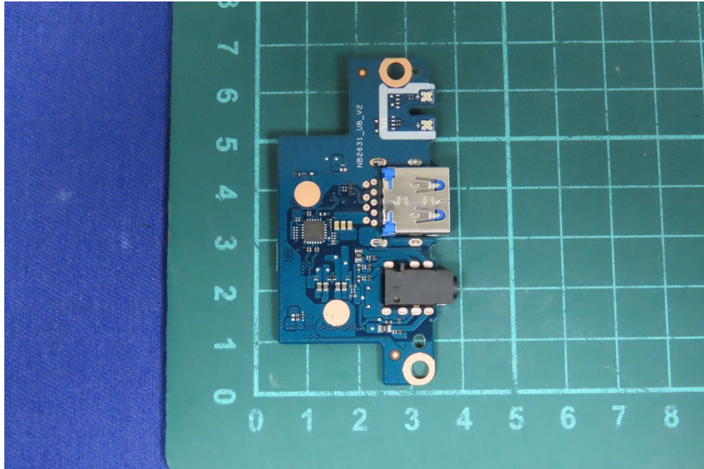
(15) EUT Photo
