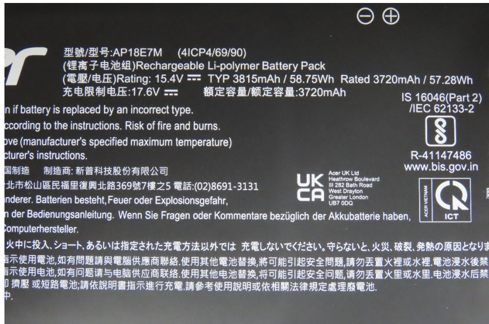
(18) EUT Photo
