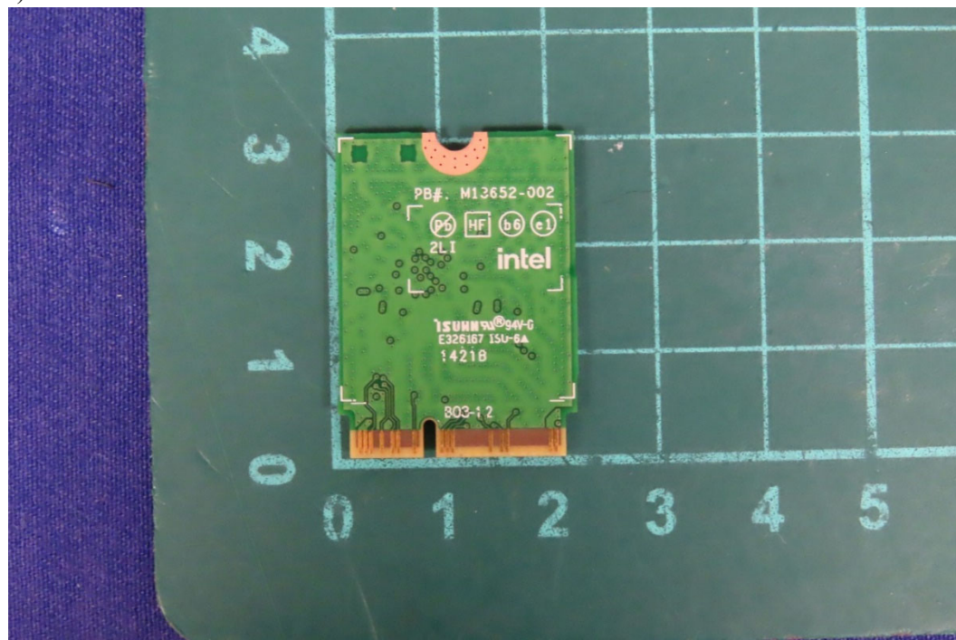
(24) EUT Photo
