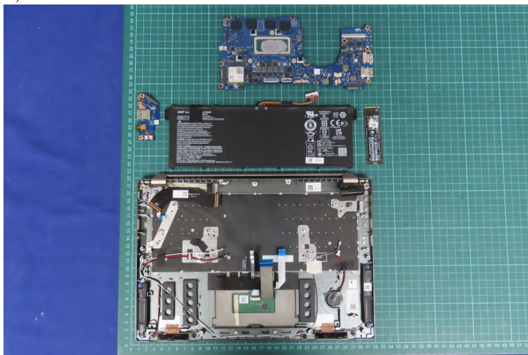
(13) EUT Photo
