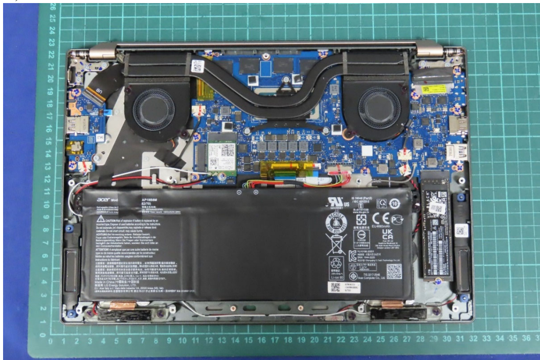
(10) EUT Photo
