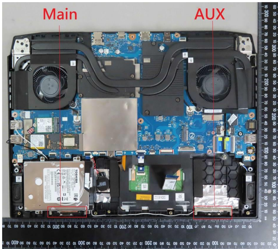
Antenna
