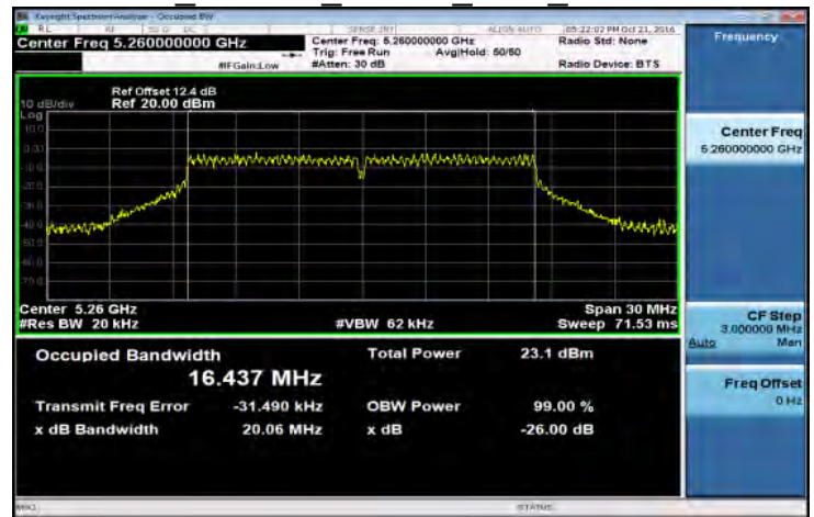
FCC 802.11a 20MHz Main 5260MHz
