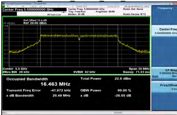
FCC 802.11a 20MHz Main 5500MHz
