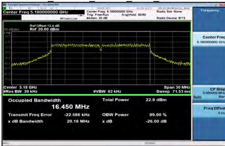
FCC 802.11a 20MHz Main 5180MHz
