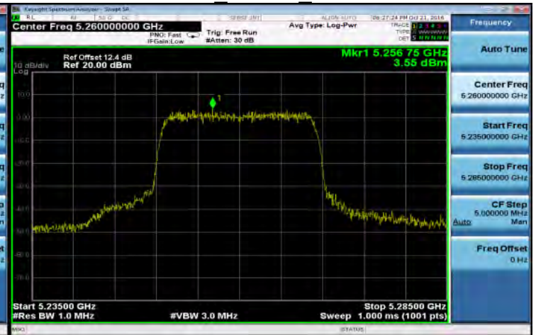
802.11n 20MHz 5260MHz
