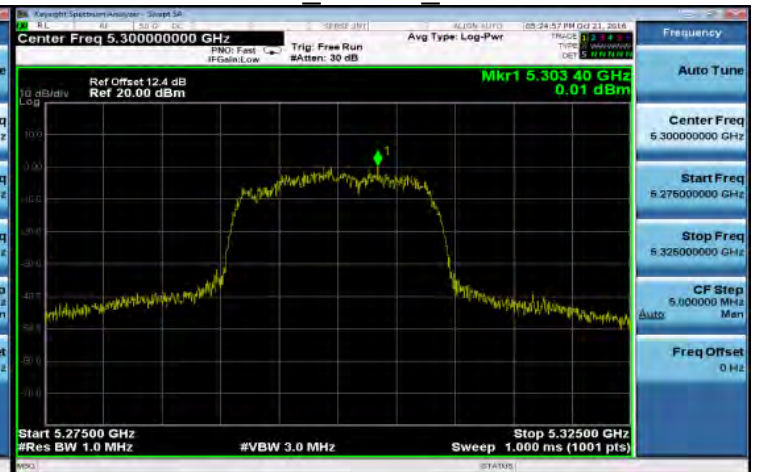
802.11a 20MHz 5300MHz
