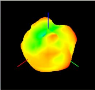
5.2G
