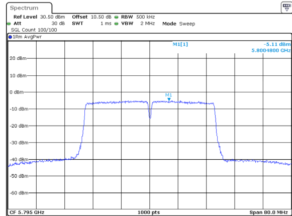
802.11ac40_5795MHz_ANT1
