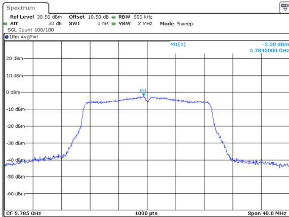
802.11ac20_5785MHz_ANT2
