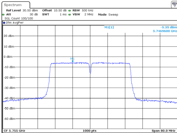
802.11ac40_5755MHz_ANT1
