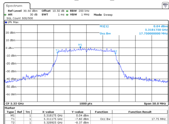
802.11ac20_5320MHz_ANT2
