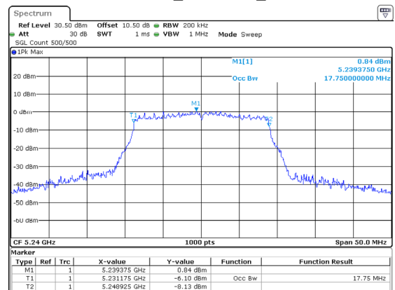
802.11ac20_5240MHz_ANT2
