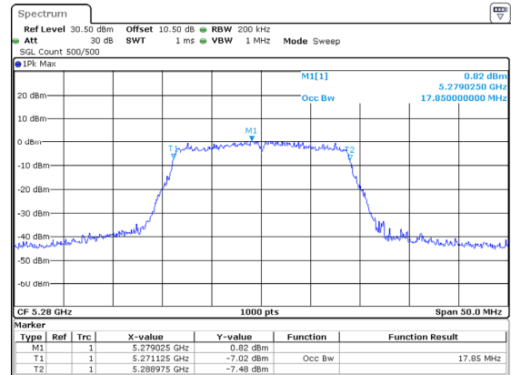
802.11ac20_5280MHz_ANT1
