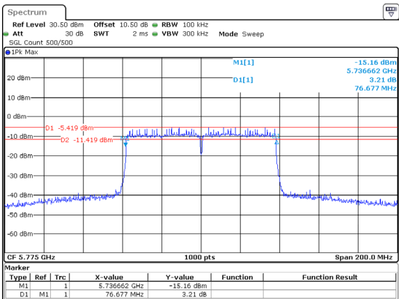
802.11ac80_5775MHz_ANT1
