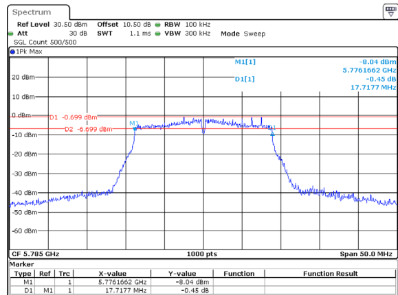
802.11ac20_5785MHz_ANT1
