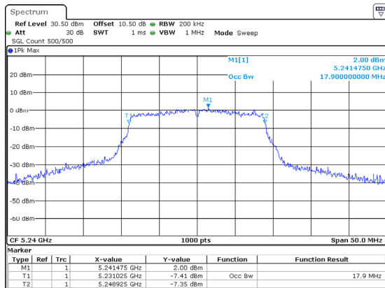
802.11ac20_5240MHz_ANT1
