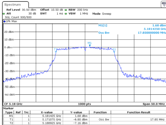
802.11ac20_5180MHz_ANT1
