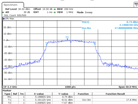
802.11ac20_5200MHz_ANT2
