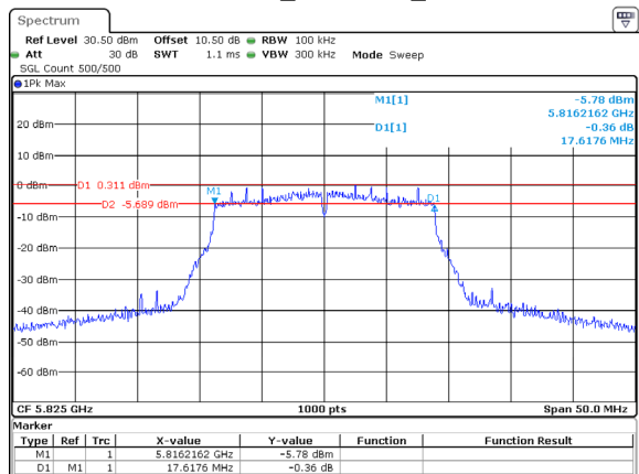
802.11ac20_5825MHz_ANT1
