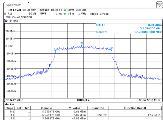
802.11ac20_5260MHz_ANT2
