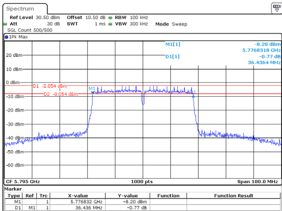
802.11ac40_5795MHz_ANT1
