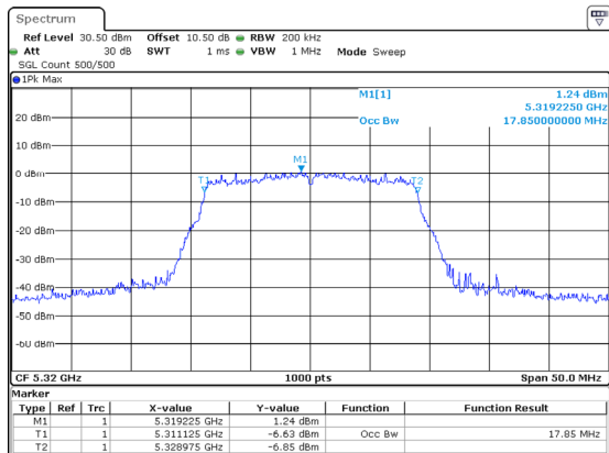
802.11ac20_5320MHz_ANT1
