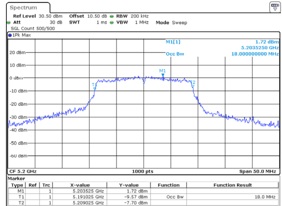
802.11ac20_5200MHz_ANT1
