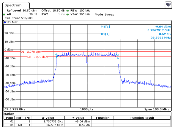
802.11ac40_5755MHz_ANT1
