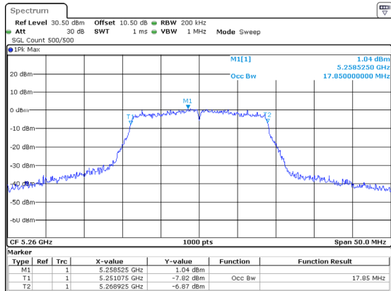
802.11ac20_5260MHz_ANT1
