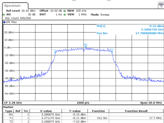
802.11ac20_5280MHz_ANT2
