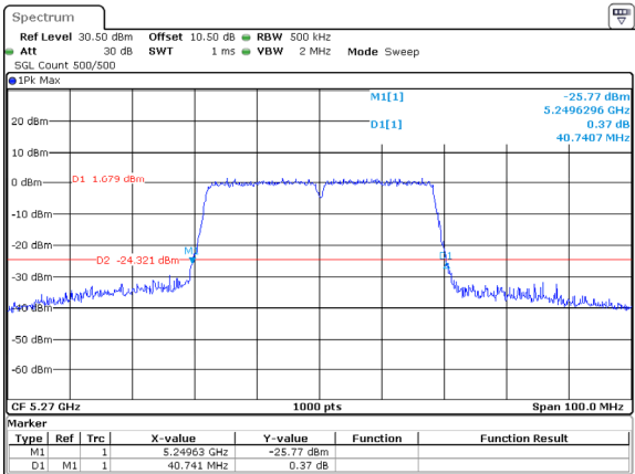
802.11ac40_5270MHz_ANT1
