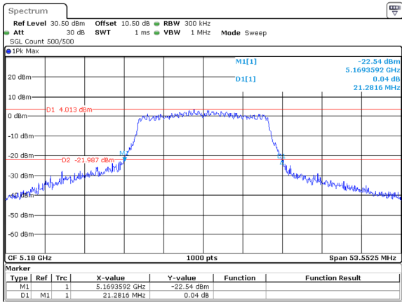
802.11ac20_5180MHz_ANT2
