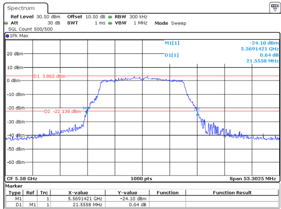
802.11a_5580MHz_ANT1
