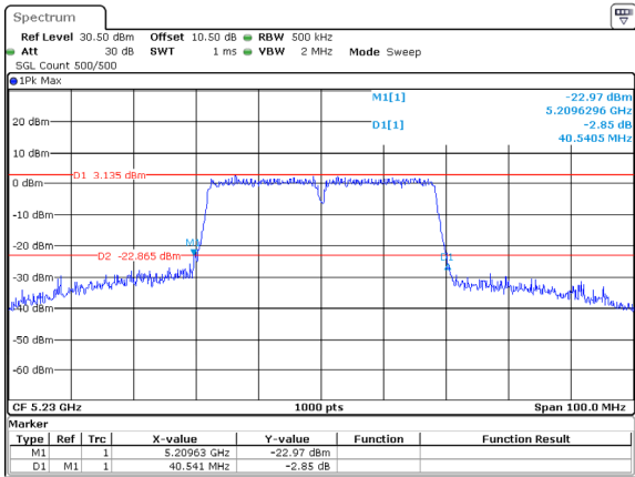
802.11ac40_5230MHz_ANT2
