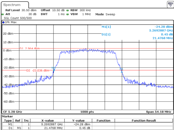
802.11ac20_5280MHz_ANT2
