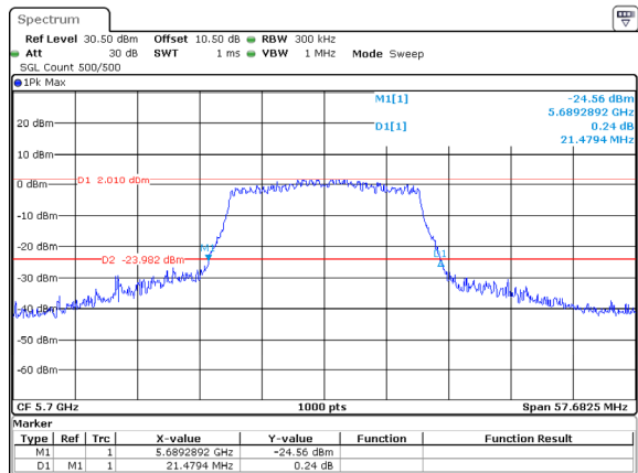
802.11ac20_5700MHz_ANT2
