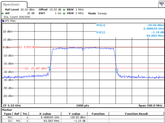
802.11ac80_5530MHz_ANT1
