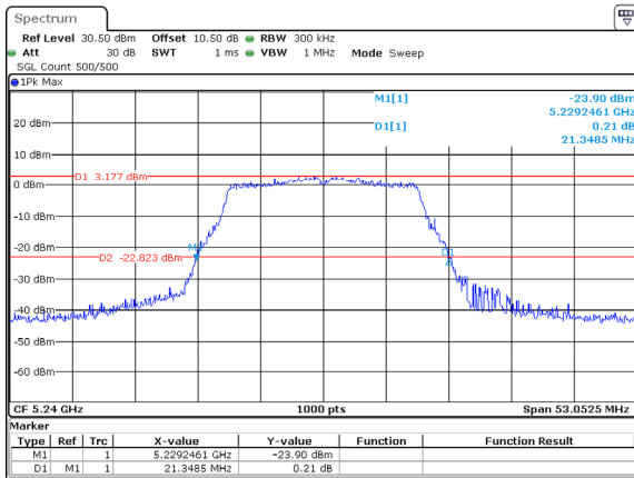
802.11a_5240MHz_ANT1
