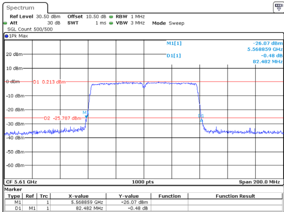
802.11ac80_5610MHz_ANT1
