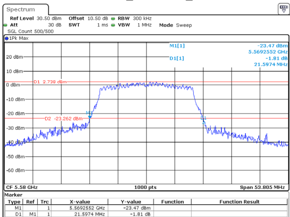
802.11ac20_5580MHz_ANT2
