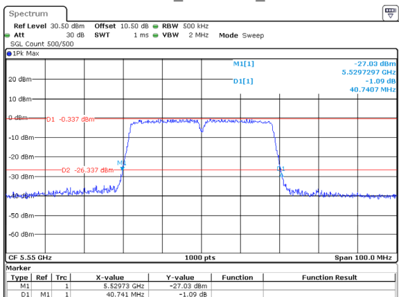
802.11ac40_5550MHz_ANT1
