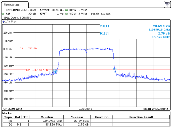
802.11ac80_5290MHz_ANT2
