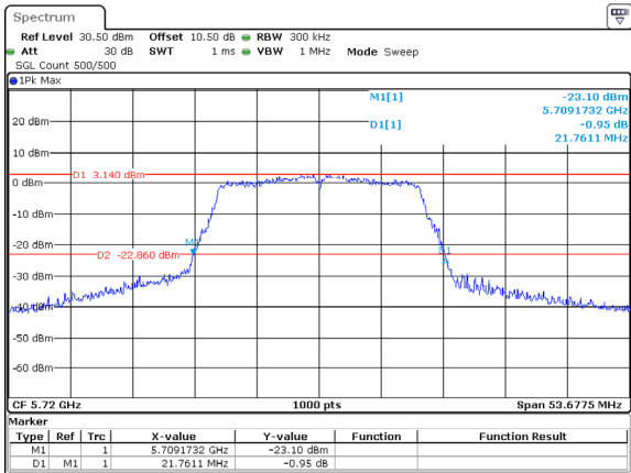
802.11ac20_5720MHz_ANT1
