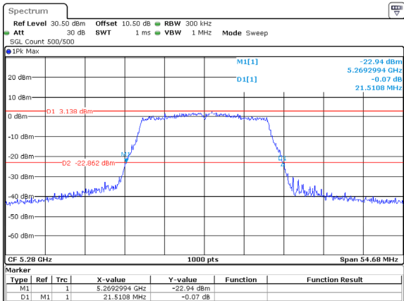
802.11ac20_5280MHz_ANT1
