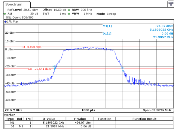
802.11a_5200MHz_ANT1
