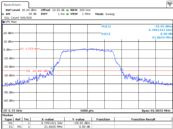
802.11a_5720MHz_ANT2
