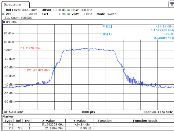
802.11a_5180MHz_ANT1
