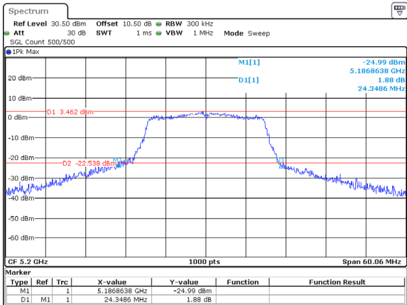
802.11ac20_5200MHz_ANT1
