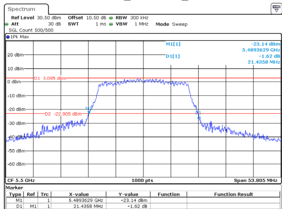
802.11ac20_5500MHz_ANT2
