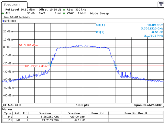
802.11ac20_5580MHz_ANT1
