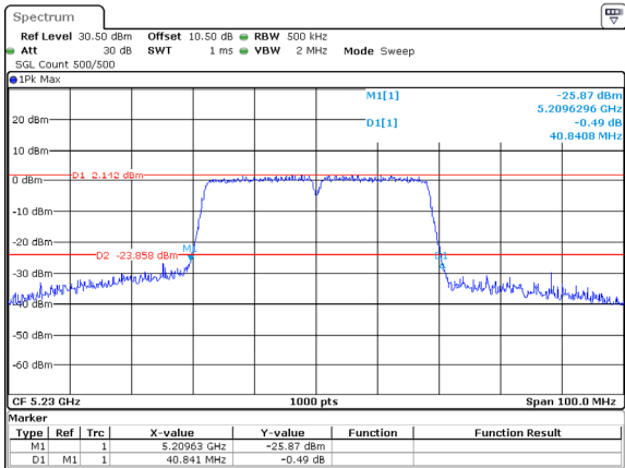
802.11ac40_5230MHz_ANT1
