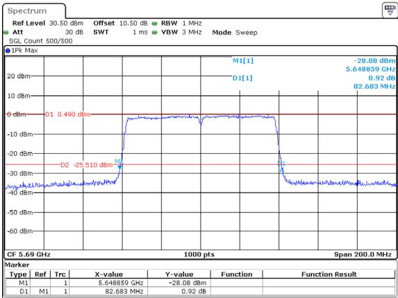
802.11ac80_5690MHz_ANT1
