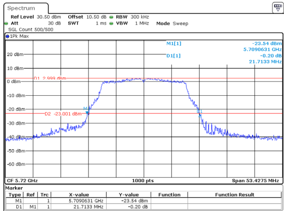
802.11a_5720MHz_ANT1
