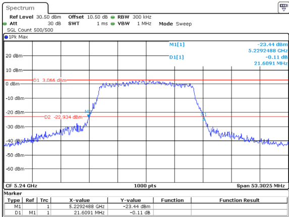
802.11ac20_5240MHz_ANT2
