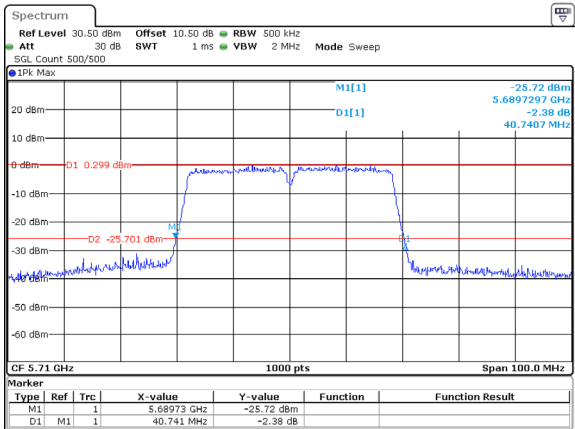
802.11ac40_5710MHz_ANT1
