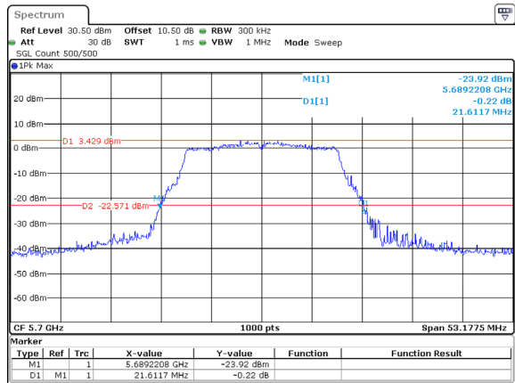
802.11a_5700MHz_ANT1
