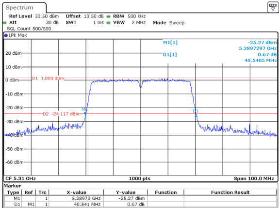
802.11ac40_5310MHz_ANT1
