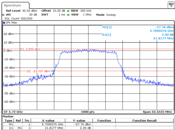
802.11ac20_5720MHz_ANT2
