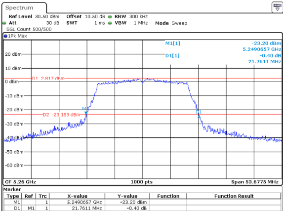
802.11ac20_5260MHz_ANT1
