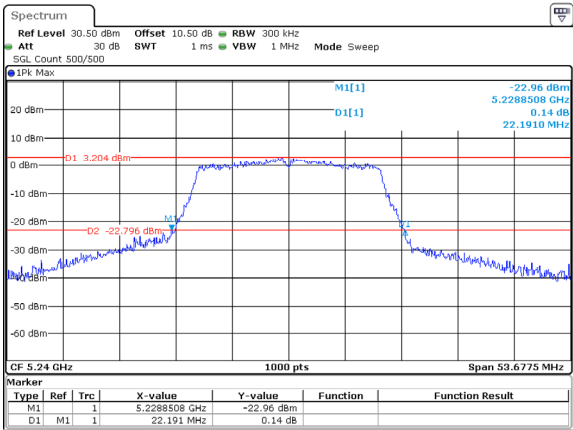
802.11ac20_5240MHz_ANT1
