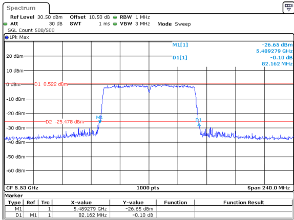
802.11ac80_5530MHz_ANT2
