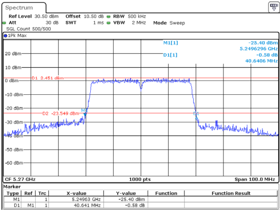
802.11ac40_5270MHz_ANT2
