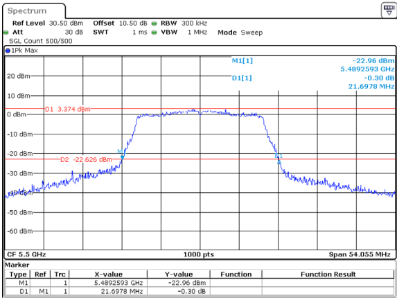
802.11ac20_5500MHz_ANT1
