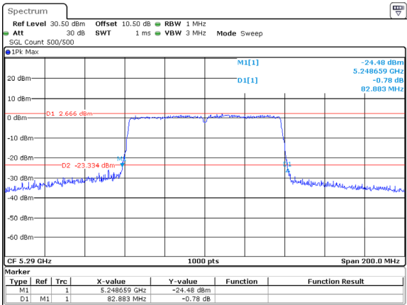
802.11ac80_5290MHz_ANT1
