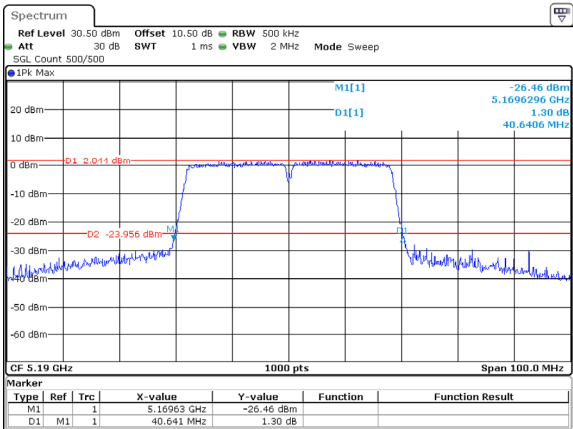
802.11ac40_5190MHz_ANT1
