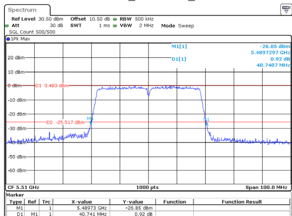
802.11ac40_5510MHz_ANT1
