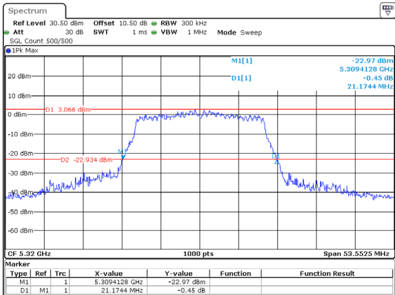
802.11ac20_5320MHz_ANT2
