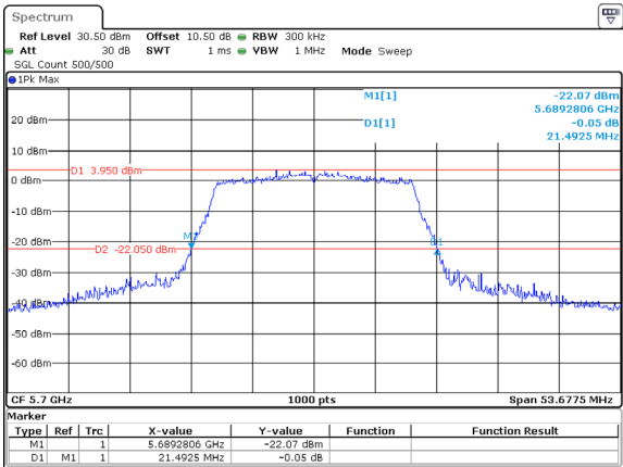
802.11ac20_5700MHz_ANT1
