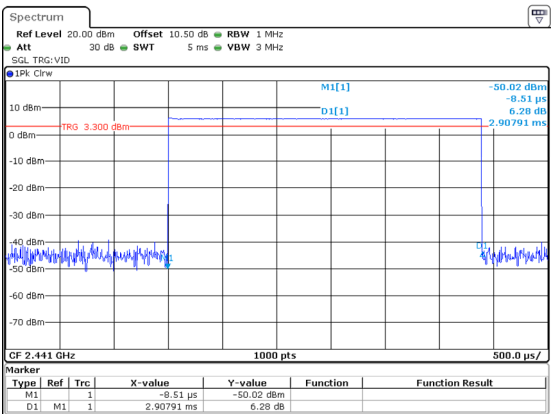
DH5_Hopping 2.908ms
