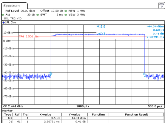
2DH5_Hopping 2.908ms
