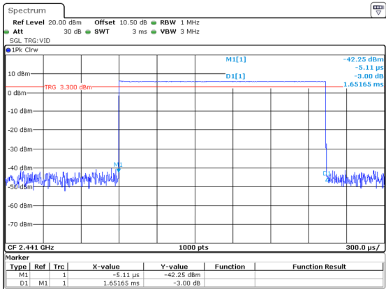
DH3_Hopping 1.652ms
