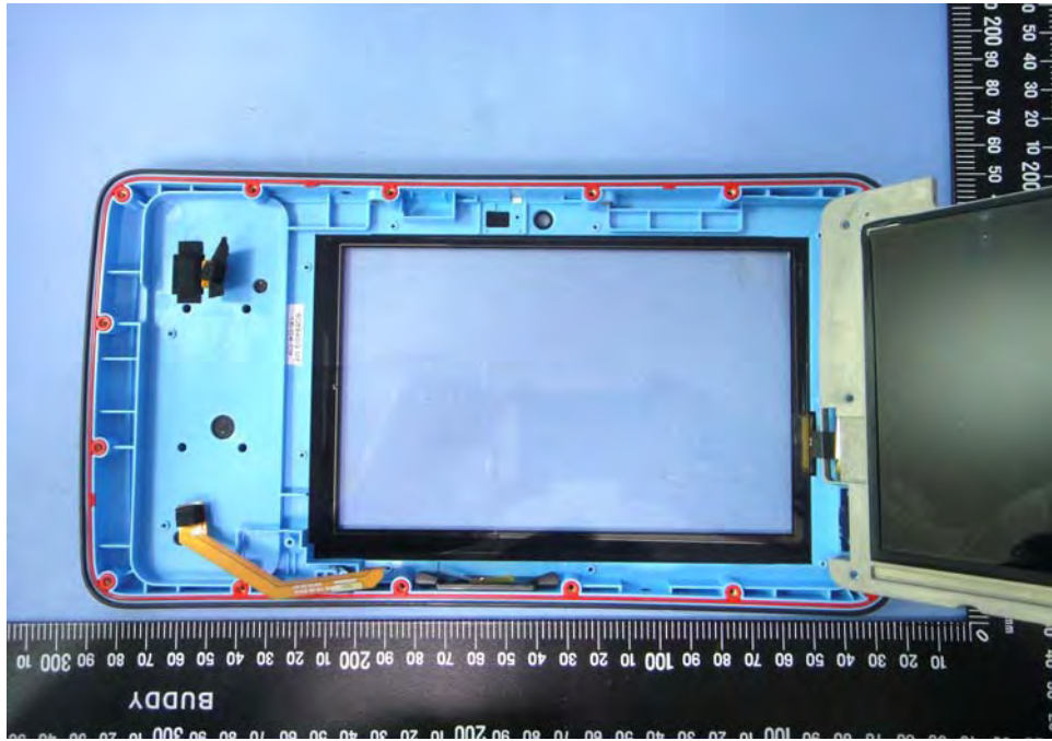
EUT Photo 33 )
