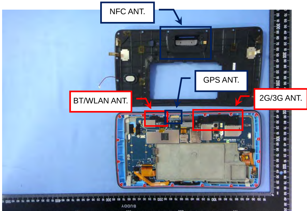
EUT Photo 6 )
