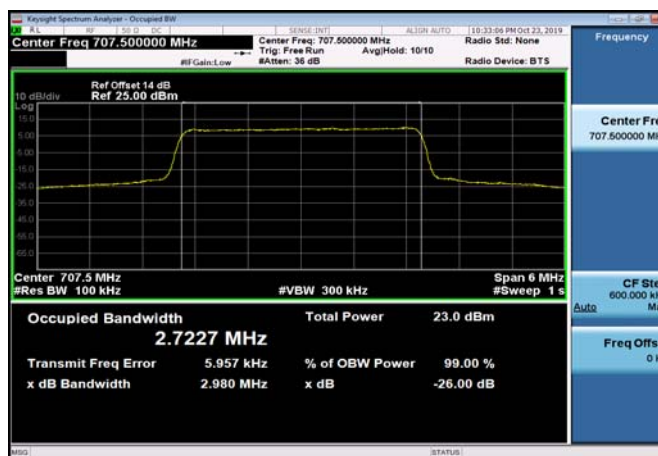
FDD12_MidRange_5MHz_707.5MHz_QPSK
