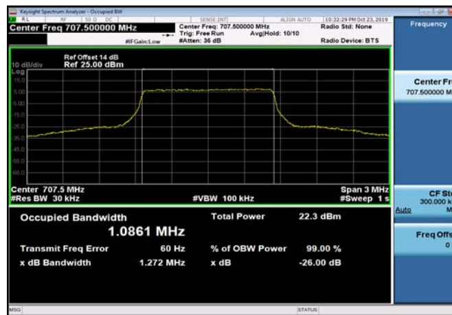
FDD12_MidRange_3MHz_707.5MHz_Q16
