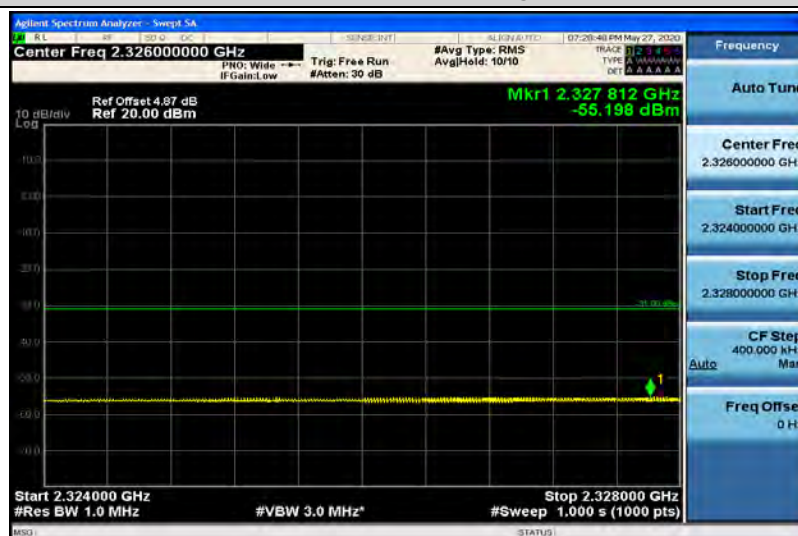
Band40-5MHz-QPSK-39225-1RB#24-Range7:2324~2328MHz
