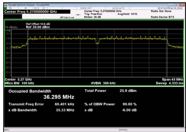
U-NII-2a 6dB Bandwidth-802.11ac(40MHz) ,5270MHz
