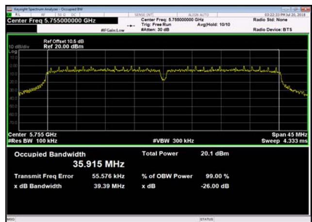
U-NII-3 26 dB Bandwidth-802.11ac(40MHz) ,5755MHz
