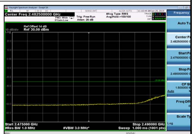
FDD07_15MHz_2507.5_Q16_fullRB_ExtraBa nds_Range_2475~2490
