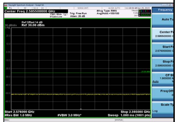
FDD07_20MHz_2510_Q16_fullIRB_ExtraBand s_Range_2576~2595
