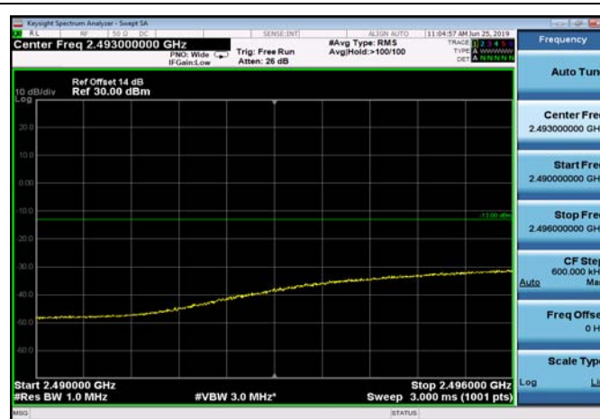
FDD07_10MHz_2505_Q16_fullRB_ExtraBand s_Range_2490~2496
