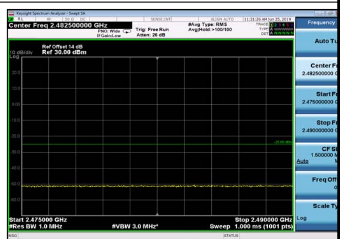
FDD07_5MHz_2567.5_QPSK_OneRB_low _ExtraBands_Range_2475~2490
