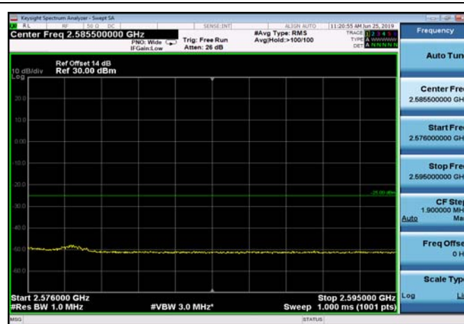
FDD07_5MHz_2567.5_Q16_OneRB_high _ExtraBands_Range_2576~2595
