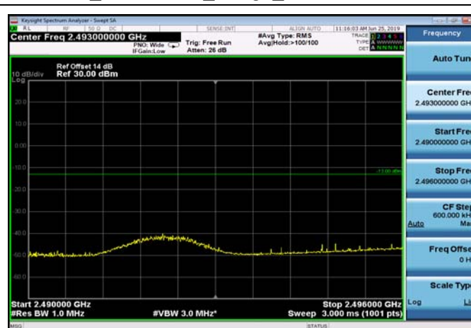
FDD07_20MHz_2510_Q16_OneRB_low _ExtraBands_Range_2490~2496
