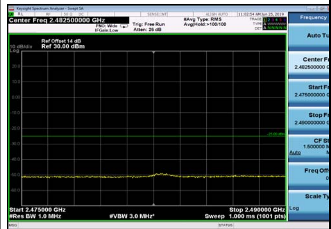
FDD07_10MHz_2505_Q16_OneRB_low _ExtraBands_Range_2475~2490
