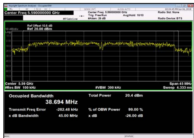
U-NII-2c -802.11ac(40MHz),5590MHz
