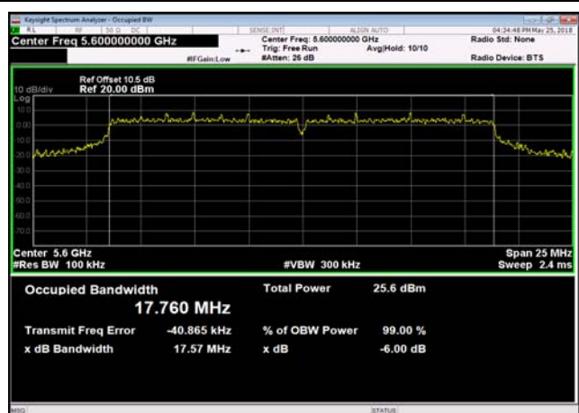
U-NII-2c,802.11n(20MHz),5600MHz
