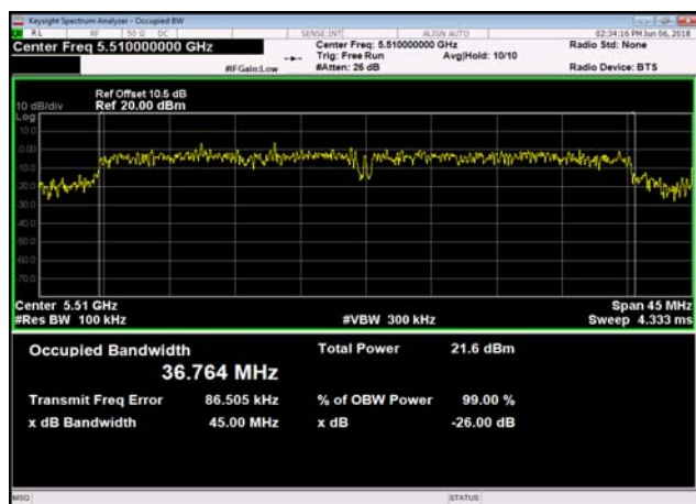
U-NII-2c -802.11ac(40MHz),5510MHz
