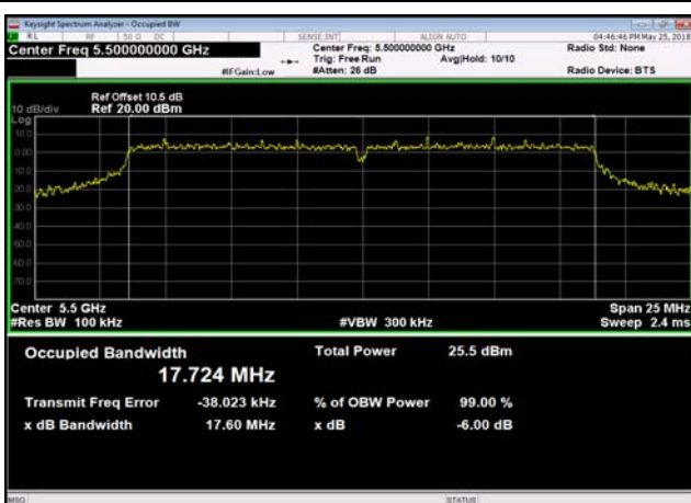
U-NII-2c,802.11n(20MHz),5500MHz
