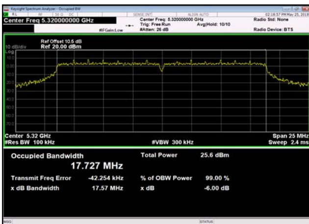
U-NII-2a,802.11n(20MHz),5320MHz
