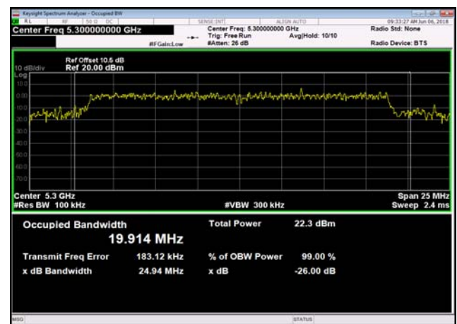
U-NII-2a -802.11ac(20MHz ) ,5300MHz
