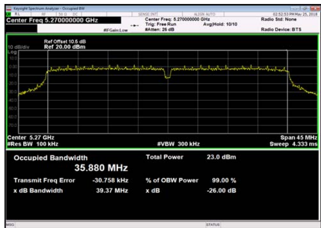
U-NII-2a,802.11n(40MHz),5270MHz
