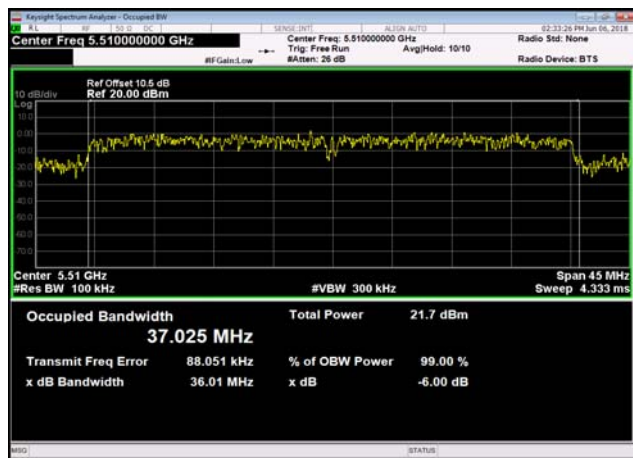
U-NII-2c 6dB Bandwidth-802.11ac(40MHz),5510MHz
