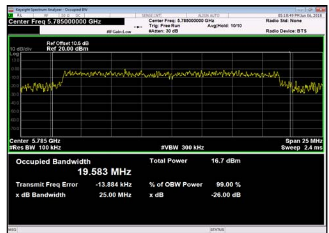
U-NII-3 -802.11ac(20MHz) ,5785MHz
