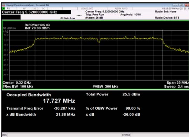
U-NII-2a,802.11n(20MHz),5320MHz
