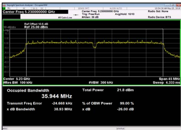
U-NII-1,802.11n(40MHz),5230MHz
