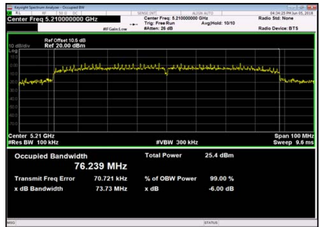
U-NII-1 6dB Bandwidth-802.11ac(80MHz) ,5210MHz
