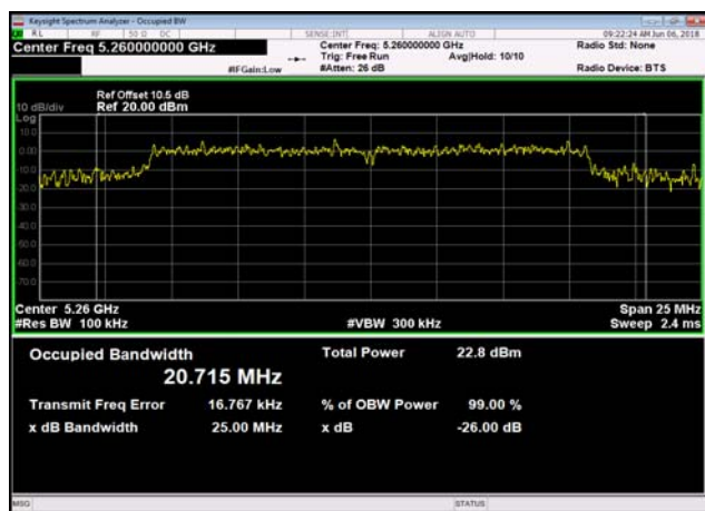
U-NII-2a -802.11ac(20MHz ) ,5260MHz
