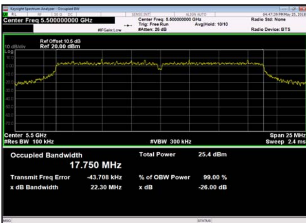
U-NII-2c,802.11n(20MHz),5500MHz
