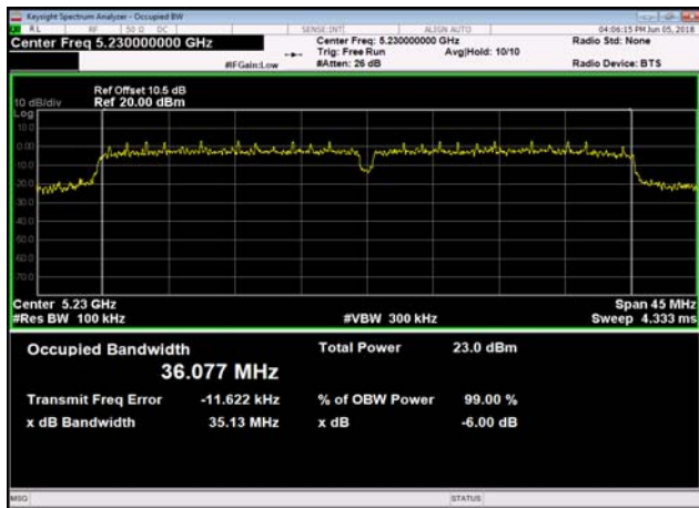
U-NII-1 6dB Bandwidth-802.11ac(40MHz) ,5230MHz
