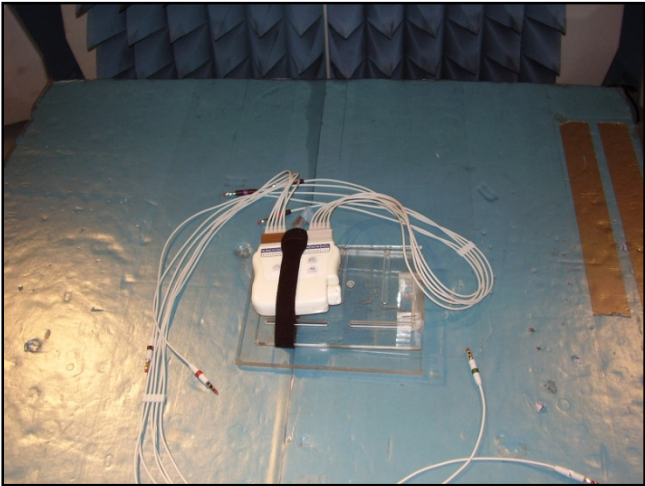
EUT Flat
