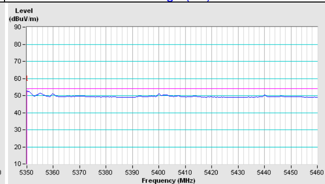
Bandedge (AV)
